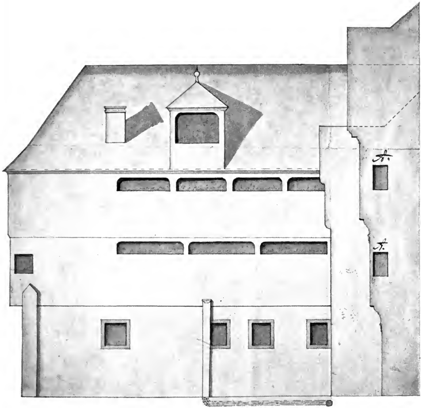
Aufriß der nördlichen Seitenfront des Goethehauses vor 1755, nebst dem Schnitt des daranstoßenden Brauhauses.
