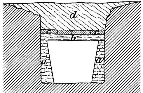
a Bruchsteinmauer. b Holzbalken. c Deckplatten. d Erde.
