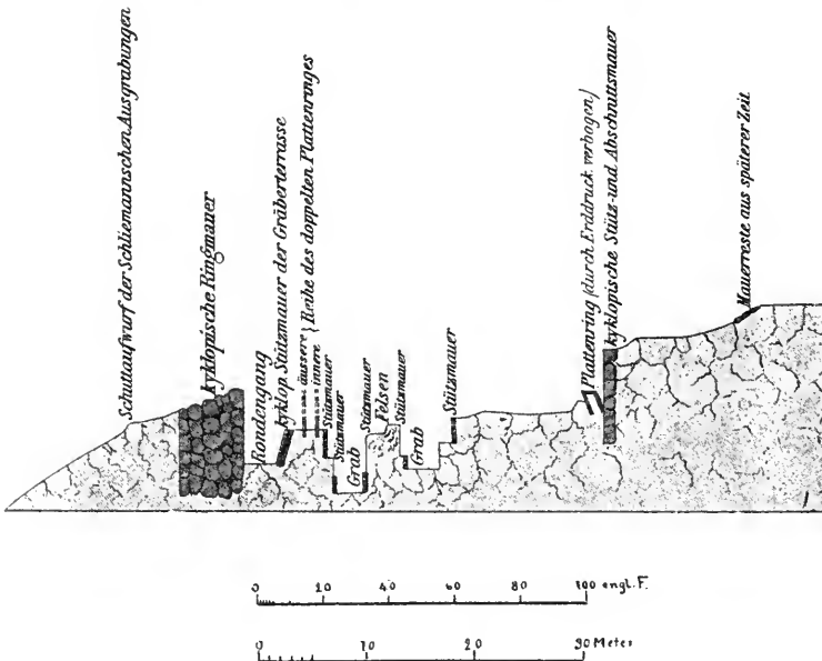
Abb. 3. Ausschnitt aus Steffens Karte der Burg von Mykene, Vertikalschnitt.
