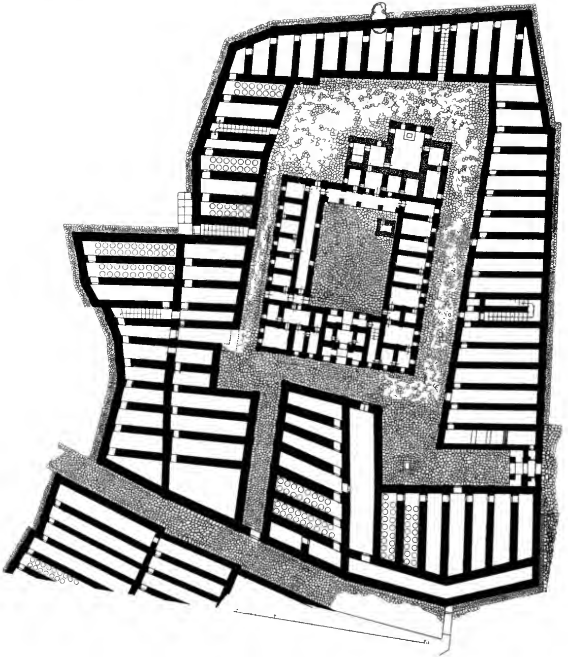
Abb. 1. Der große Tempel von Boghasköi mit den vielen, ihn rings umgebenden Magazinen. Rekonstruierter Grundriß in 1 : 1000. Orientierung S. 41° W.
