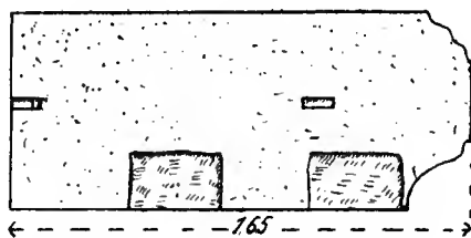
Abb. 7. Ein Epistyl der neronischen Bühne in Oberaufsicht (Obergeschoß).
