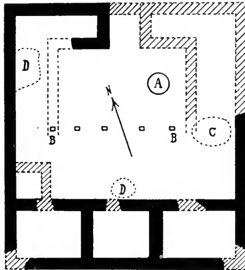
Abb. 13. Prätorium des Kastells Melandra. (A Grube oder Brunnen [darin oberer Teil eines Altars]. B Holzpfosten. C Nicht ausgegraben. D Steinpflaster.)
