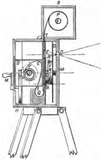
Fig. 115. Längsschnitt durch den Kinematograph.
