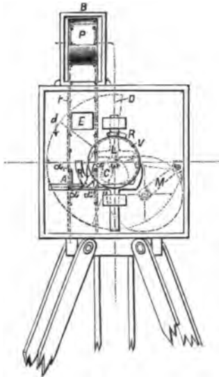
Fig. 116. Vertikaler Querschnitt.
