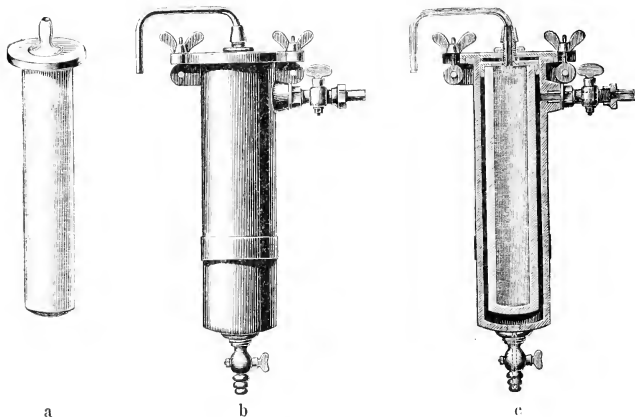
Kieselguhrfilter System NORDTMEYER-BERKEFELD.
