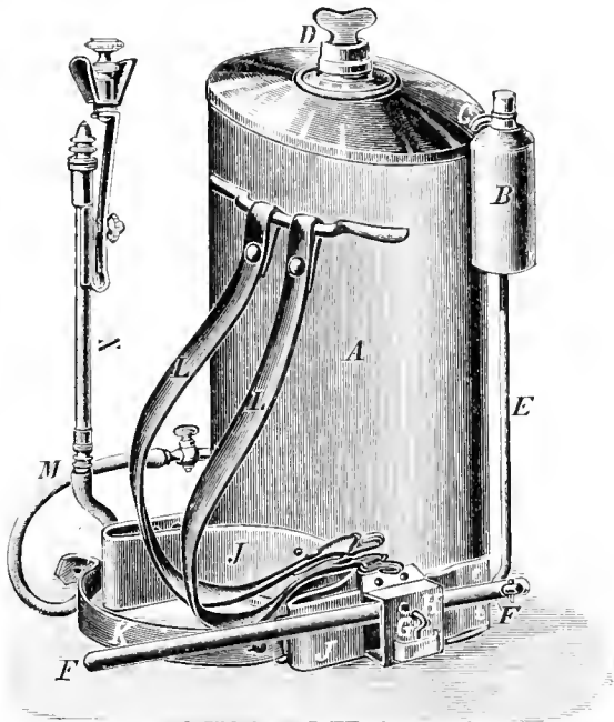
Universalspritze „Saxonia“. Von G. Drescher-Halle a. S.
