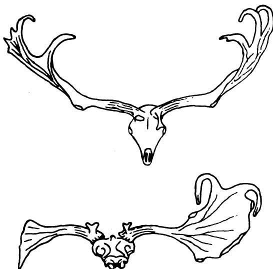
Fig. 2. Cervus (euryceros) Germaniae Pohlig (Typusexemplare der Germaniar- | Rasse). Ansicht der Bonner Geweihe von oben und von hinten. Kopie nach Pohlig, l. c. fig. 3. ca. \frac{1}{21} nat. Gr.
