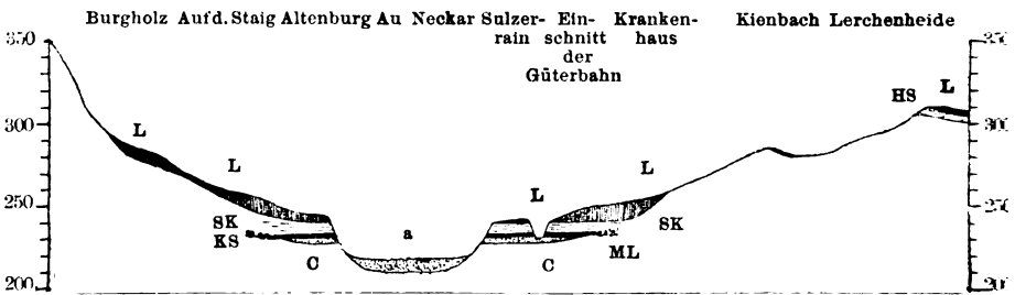
Profil durch das Cannstatter Talbecken von WNW nach OSO, vom Bahnhof zur Lerchenheide. Maßstab für Höhe 1 : 5000; für Länge 1 : 50 000.
