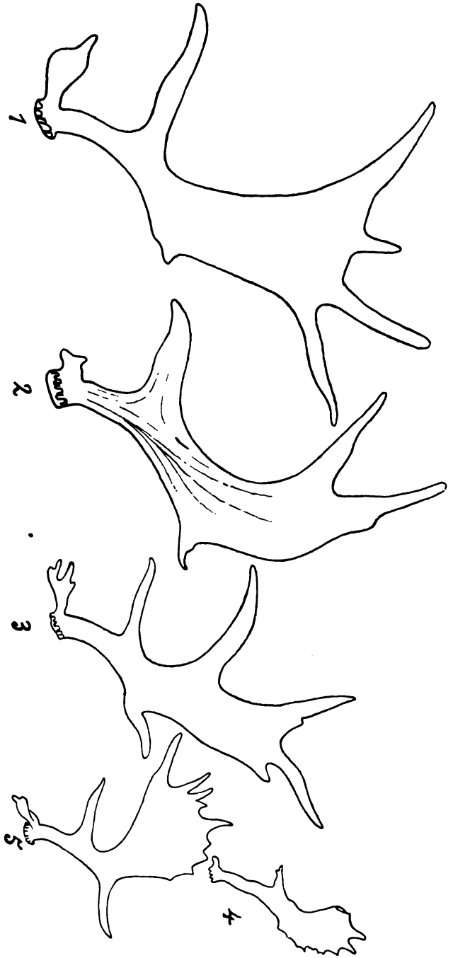
Fig. 1. Ansicht verschiedener deutscher Riesenhirschaufeln von innen.
