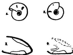
Fig. 7. Schmelzleisten von Pl. (Segm.) Lartetii NOULET.
