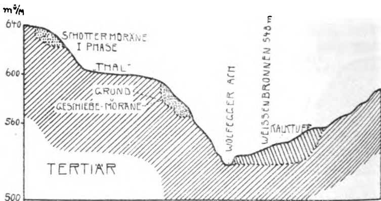
Abb. 4. Querschnitt durch das Wolfegger Aachtal bei Weißenbronnen.
