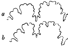
Fig. 1. Amm. convolutus exesus . Original zu QUENSTEDT'S Amm. d. schwäb. Jura Tab. 81 fig. 16. a vorletzte Lobenlinie. b sechstletzte Lobenlinie. 3fach vergr.
