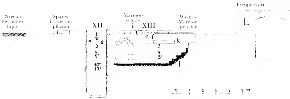
Fig. 95 Schnitt durch die nordöstliche Hälfte des Comitiums. Vgl. den Plan Fig. 78.
