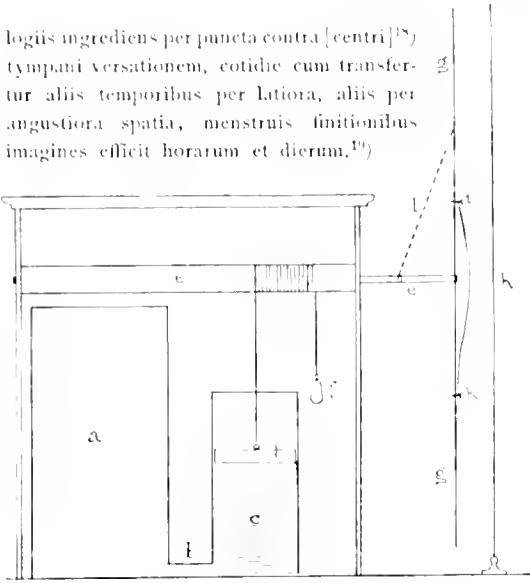
Fig. 22 Längsdurchschnitt der astronomischen Uhr nach Vitruv und dem Salzburger Fragment.
