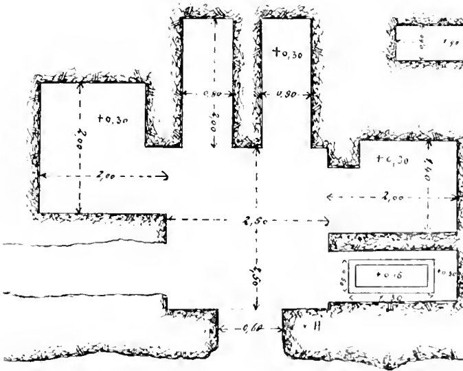
Fig. 31. Horizontālschnitt durch Grab C.
