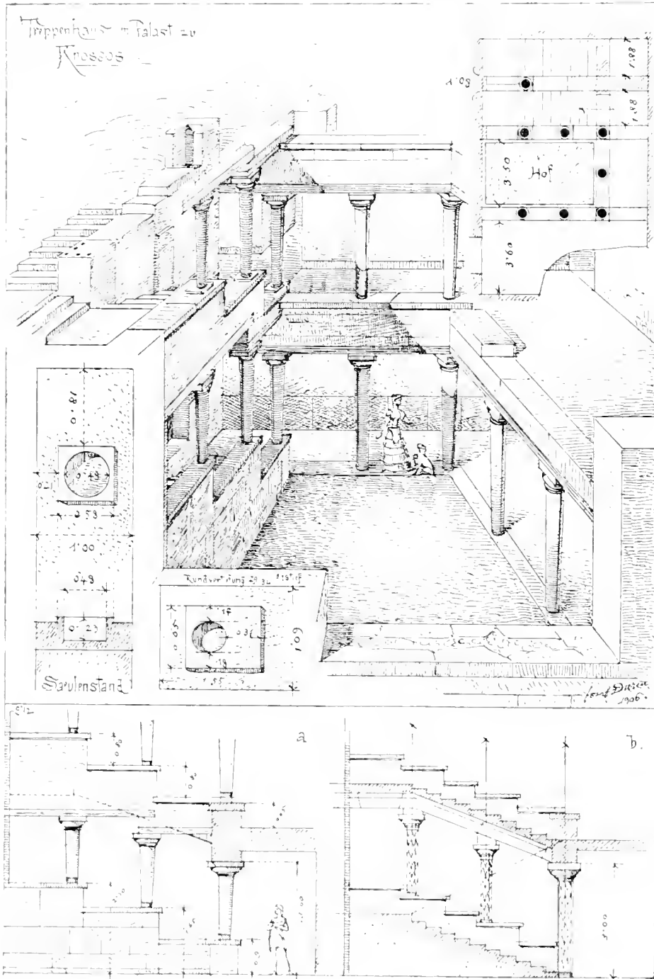
39: Treppenhaus im Palast zu Knossos.
