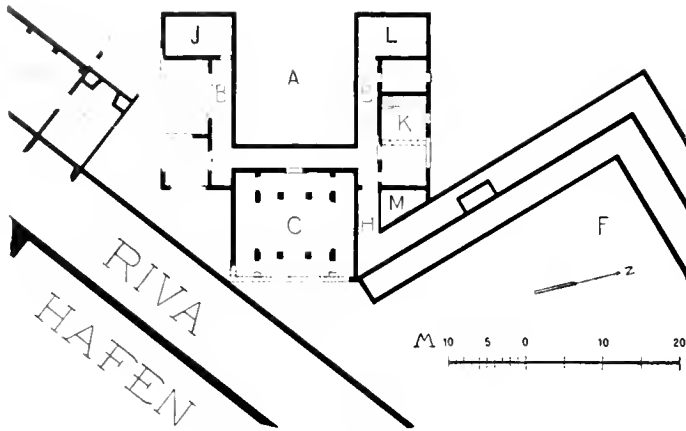
3: Grundriß der Diæta zwischen Porticus und Palaestra.
