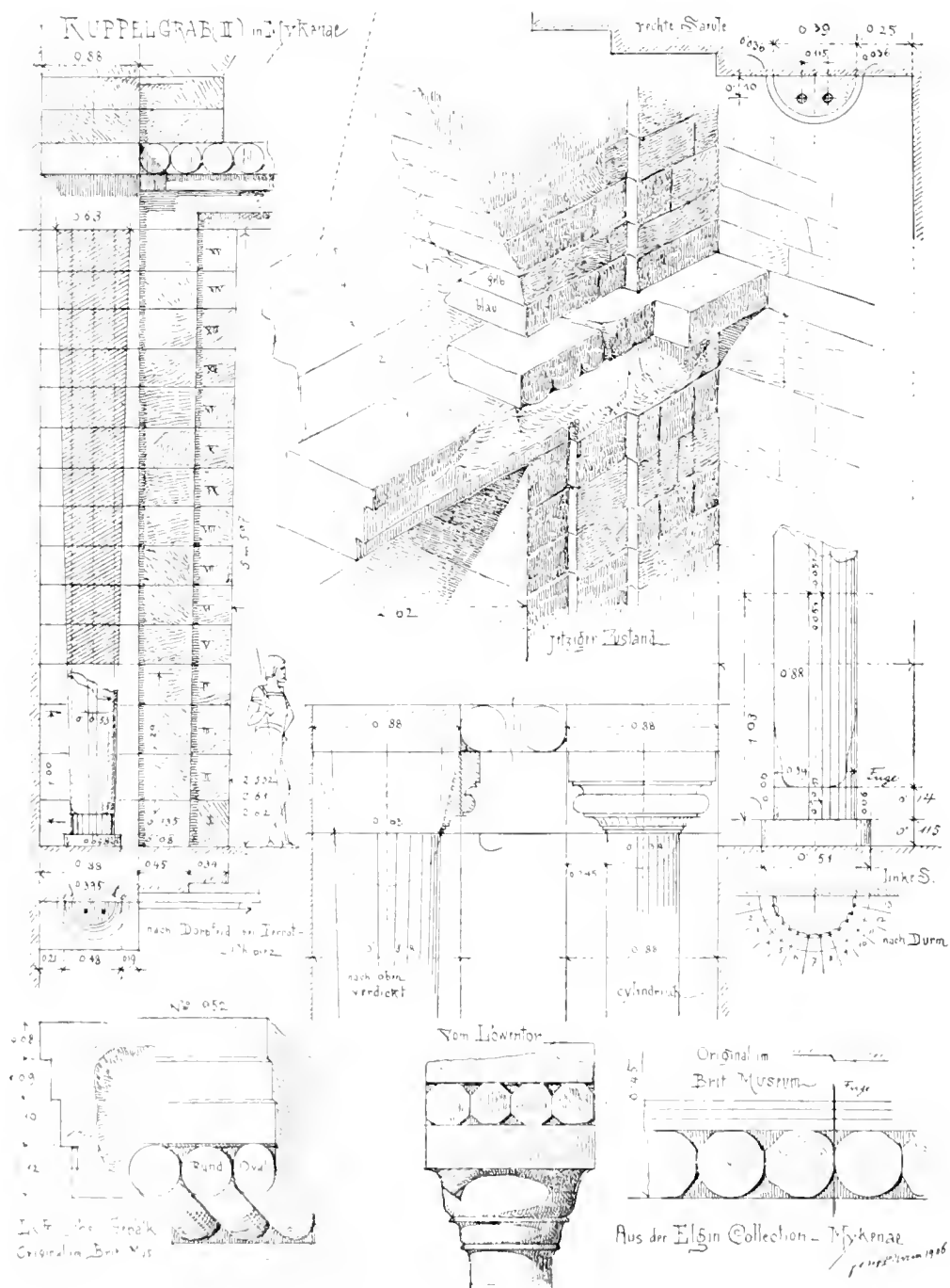
17: Vom zweiten Kuppelgrab in Mykenai.
