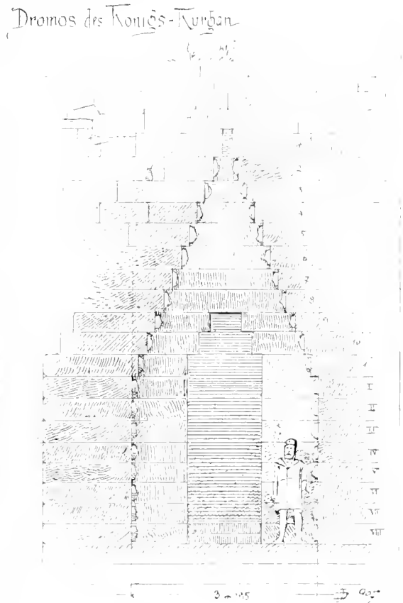
76: Querschnitt des Dromos des Königs-Kurgans.
