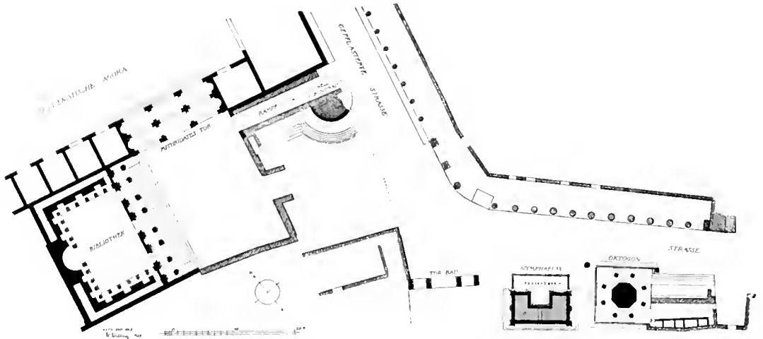
9: Grundriß der Bibliothek und der angrenzenden Bauten.
