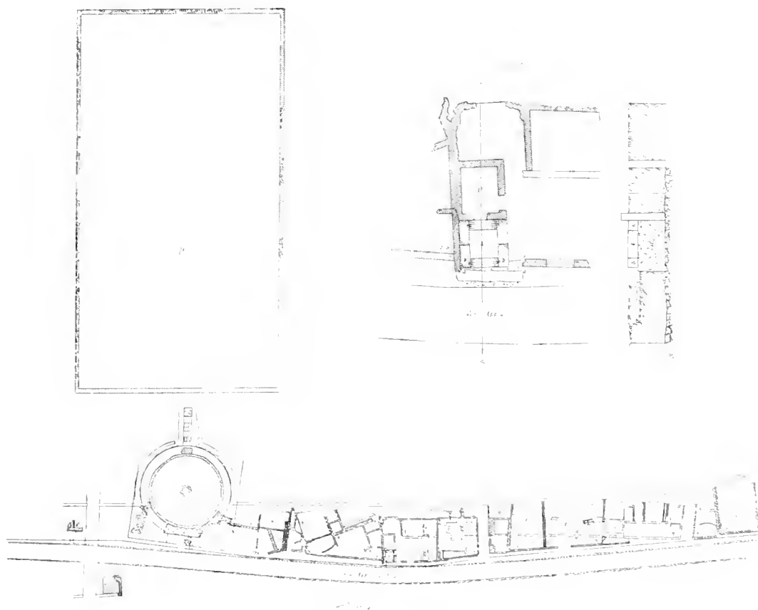
59: Planimetrie del gomito stradale al V o miglio con particolari e sezione del monumento 1.
