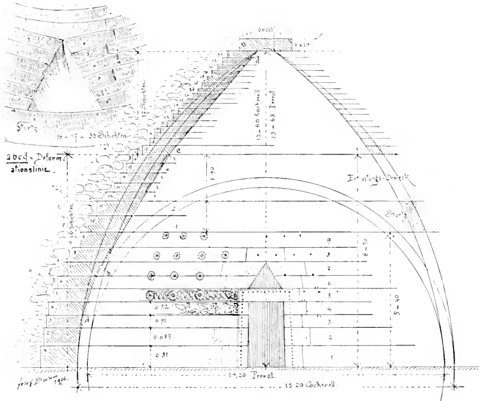
23: Querschnitt der Atræustholos in Mykenai.
