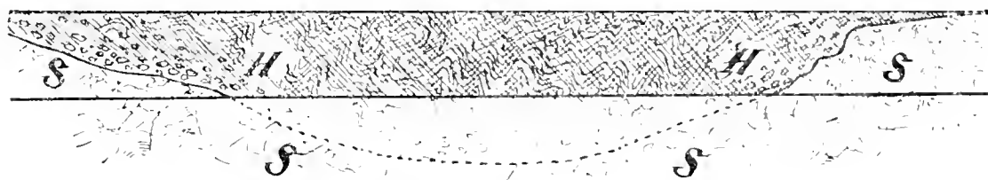
Fig. 5. Einsenkung der stark gefalteten, sehr festen Anhydrite im Hangenden ( H ) in das Salzlager ( S ). Seitliche (uördliche) Versuchsstrecke von der Strecke West No. 4. Massstab 1:100.
