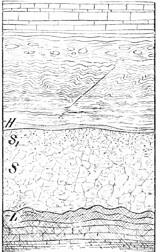
Fig. 6. Profil durch das Salzlager von Wilhelmshluck 1 : 200. S = Steinsalz, S 1 = körniges Salz, L = Liegendes einen stark welligen Boden bildend, aber nach unten in die glatten Orbicularis -Bänke übergehend. H = Hangendes, Decke von festem Anhydrit, darüber dünnbankiger, gefalteter Anhydrit, oben schlieriger Anhydrit und schliesslich wohlgeschichtete ebene Bänke von Anhydrit.
