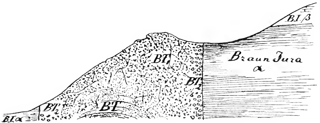
Fig. 1. Profil durch den Vulkan-Punkt im Mollenhof von Süd nach Nord. — B.I.α = Braun-Jura α ( Opalinus -Thone). B.I.β = Braun-Jura β (Personaten-Sandstein). BT = fester Basalttuff mit viel Basalt in Form kleiner Thränen (Thrärentuff). BT 1 = lockerer typischer Basalttuff. BT 2 = Mantel von Weiss-Jurabreccie mit Basalttuff.
