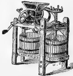
BUCKEYE CIDER MILL.
