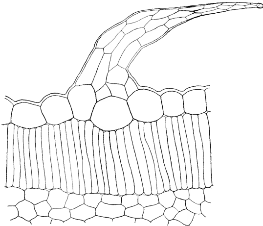
Fig. 2. — Poil pluricellulaire de la feuille de Cuphea antisiphilitica H. B. K. (Gr. = 350.)
