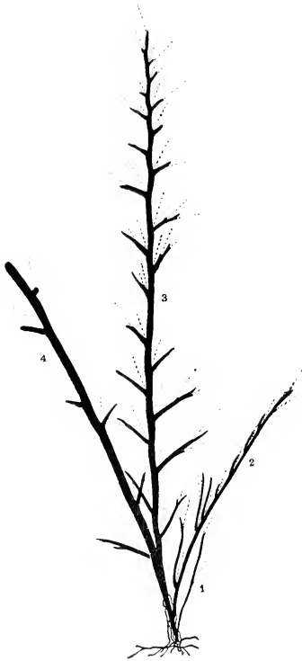
Fig. 9. — Hal. scoparia Sauv. — Une plantule de même âge que celles de la figure 8, mais composée de quatre générations de pousses indiquées par les chiffres 1, 2, 3, 4. (Gr. 12.)
