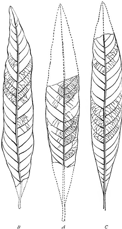
Fig. 9. — Pasianopsis vittatus Sap. et Mar., red. de 1/3. A. Feuille de Gelinden (type de l'espèce). B. Feuille de Belleu, légèrement enroulée sur les bords (type du Salix deperdita Wat.). C. Feuille de Belleu (type du Salix crebrinervia Wat.) B, C, Coll. Museum de Paris.
