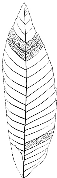
Fig. 7. — Dryophyllum subcretaceum Sap. (type du Carpinus suessionensis de Wat.), réél. (coll. Museum de Paris).
