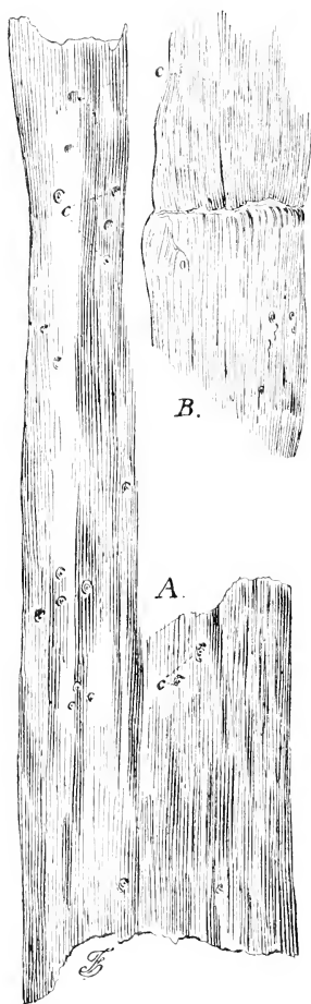
Fig. 3. — Lambeau de ? tige du Rhizocaulon eocenicum Watt. sp. En c , cicatrices radicales. Grandeur naturelle. — B . Tige du Rhizocaulon macrophyllum Sap., d'après la figure de Saporta. Très réduit.
