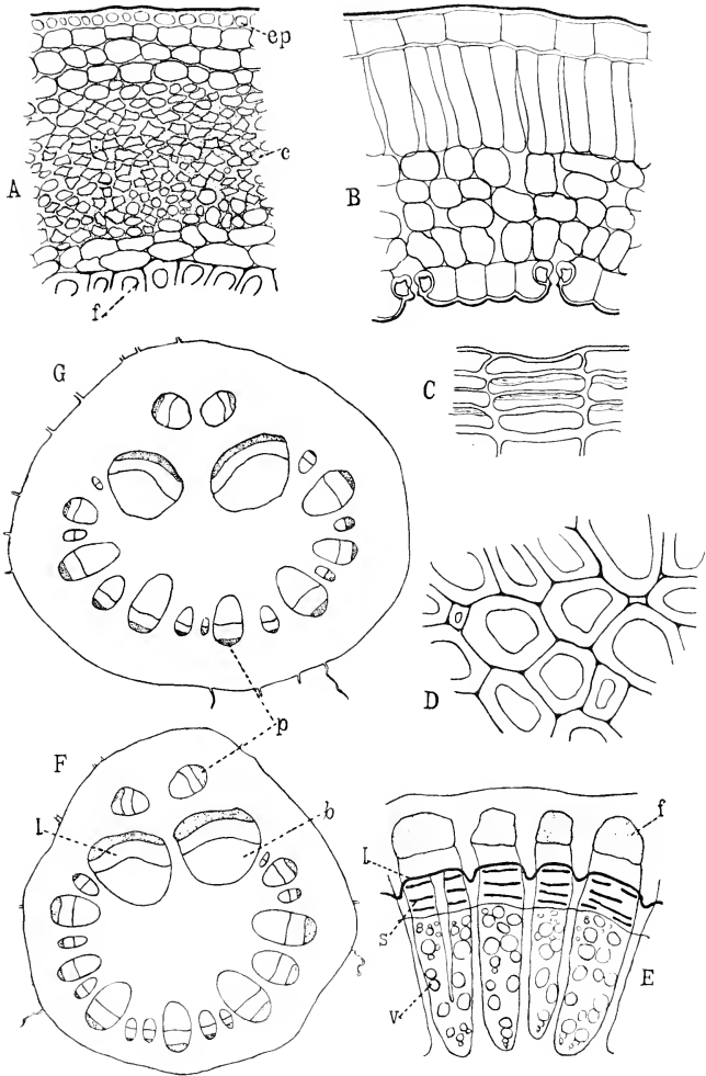
Fig. 2. — Vitis aestivalis Michaux ; mêmes lettres.
