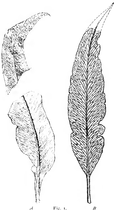
A. Fronde du Taenites crassicosatus Wat. sp., d'après les types (coll. Mus. Paris). Grandeur naturelle. B. Fronde stérile du Taenitis blechnoides Sw. actuel de l'Asie tropicale. (Herb. Mus. Paris). Réd. 1/4.
