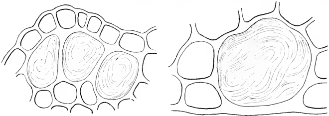
Fig. 4. — Epiderme de la feuille de Lagerstræmia villosa Wall. avec cellules à mucilage. (Gr. = 350.)
