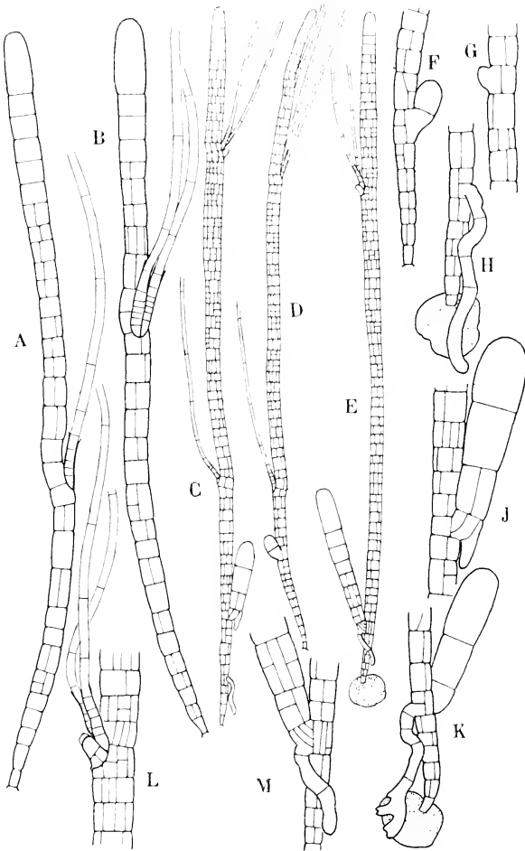
Fig. 4. — Hal. scoparia Sauv. — A, B , Plantules de la même récolte que celles de la figure 3; B , l'un des deux filaments dressés du disque H (fig. 3) porte deux poils géminés. (Gr. 150.) — C à M , Plantules obtenues le 1 er mars de déhiscences du 6 janvier. — C, D, E , Filaments entiers montrant le début des pousses de seconde génération. (Gr. 100.) — F à M , Portions de filaments, plus grossies, montrant l'insertion des pousses de seconde génération, ou les rhizoïdes, ou l'insertion des poils. (Gr. 150.) — Le disque est indiqué par un pointillé sur E, H, K .
