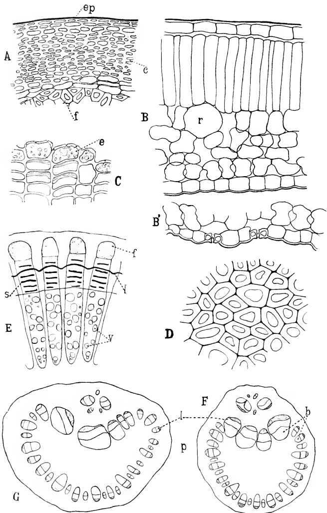
Fig. 1. — Vitis Lincoecumii Buckley. — A , partie externe d'une branche moyenne d'un an; ep , épiderme; c , collenchyme; f , fibres péricycliques (G : 150). — B , limbe en coupe transversale; r , cellule à raphides (G : 300); B' , épiderme de la face dorsale avec stomates (G : 300). — C , cellules du liège en coupe transversale; quelques-unes offrent des épaississements de nature pectique (G : 300). L'assise externe e est formée d'éléments lignifiés-ponctués. — D , quelques fibres péricycliques de la tige en section transversale (G : 300). — E , schéma d'une portion de la section transversale d'un entre-nœud; f , faisceau de fibres péricycliques; l , périderme; s , strates tangentielles de fibres libériennes; v , vaisseaux ligneux (G : 15). — F , section transversale du pétiole au 1 er tiers; G , au 2 e tiers, à partir du point d'incursion sur la tige; b , bois; l , liber; p , fibres péricycliques (G : 12).
