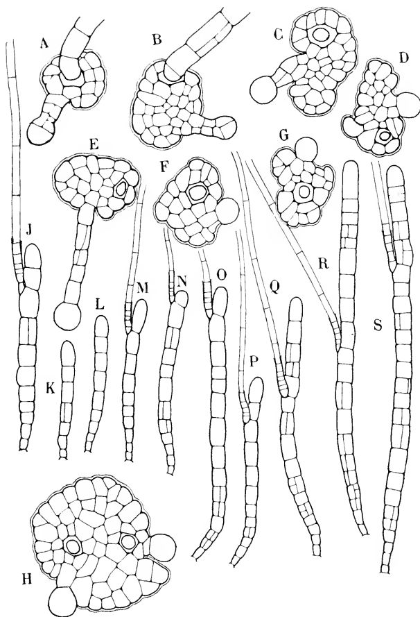
Fig. 3. — Hal. scoparia Sauv. — Plantules obtenues à Banyuls, le 20 février, de déhis- cences du 6 janvier. — A à H, Disques rampants; la base du filament dressé est dessinée sur A et B; son insertion est seulement indiquée sur C à H; H est formé par la soudure de deux disques. (Gr. 360.) — J à S, Jeunes filaments dressés à divers états de développement. (Gr. 150.)
