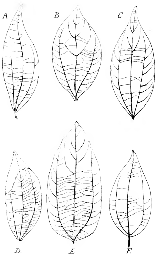
Fig. 15. — Cinnamomum Lorteti Wat. et ses variétés.
