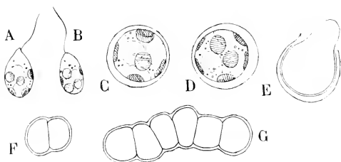
Fig. 1. — Hal. scoaria Sauv. — A, B , Zoospores en mouvement. — C, D , Zoospores fixées, entourées d'une membrane inégalement épaissie. — E , Début d'une germination. — F, G , Zoospores fixées, contiguës. (Grossissements divers, d'après des croquis pris sur le vivant.)
