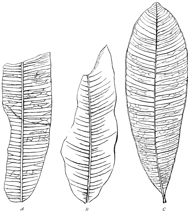
Fig. 20. — Apocynophyllum cenomanense Crié.
