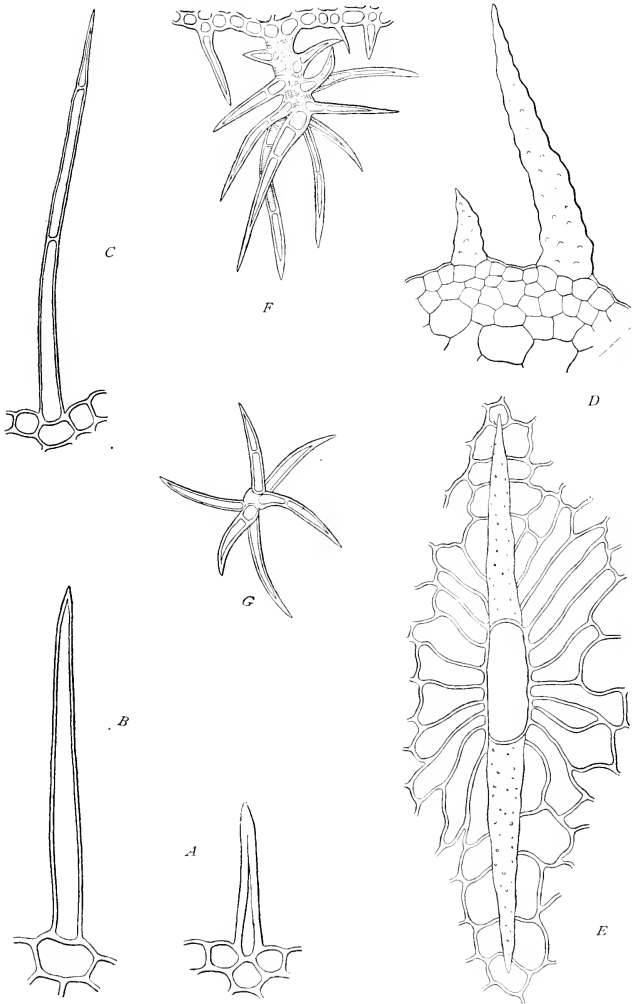
Fig. 3. — A, B, C , poils simples de Lagerstramia villosa Wall.; D, E , poils ramifiés de Lagerstramia Londoni Teysm.; F, G , poils en navette de Cuphea Llavea Lindl. (Gr. = 350).
