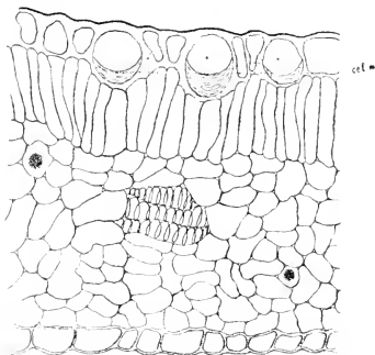
Fig. 3. — Coupe d'une feuille de P. edulis .
