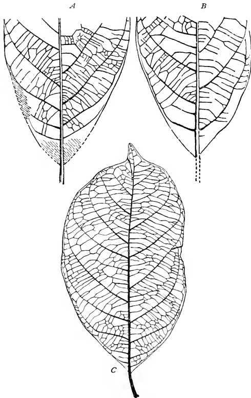
Fig. 13. — A, B. Artocarpidium Desnoyersi Wat. Bases de feuilles du grès de Belleu, réd. de 1'3. C. Artocarpus integrifolia Linn., des Indes orientales, réd. de 1'3.
