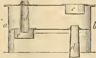
Fig. 19. — Tronçon et plateau de la colonne distillatoire.
