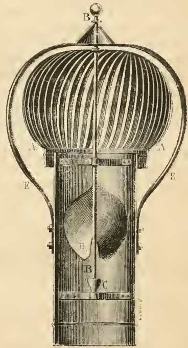
Fig. 68. — Vue du ventilateur à hélice de M. Serron. Fig. 69. — Coupe du ventilateur à hélice.
