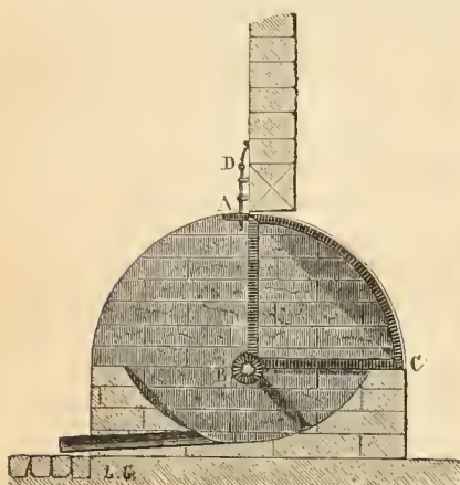
Fig. 75. — Coupe verticale d'une auge à pores fermée par un volet cylindrique.
