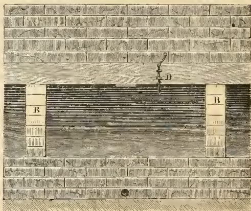
Fig. 76. — Vue de face d'une auge à pores fermée par un volet cylindrique.
