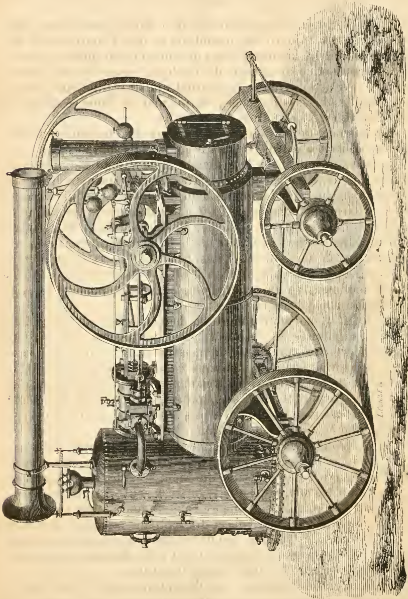
Fig. 32. — Locomobile Gérard, de Vierzon.
