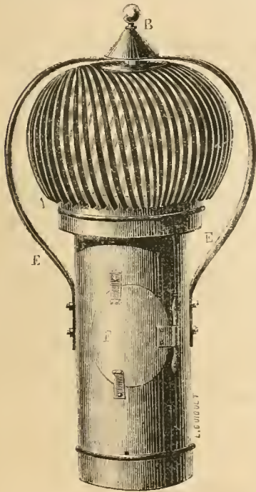
Fig. 68. — Vue du ventilateur à hélice de M. Serron. Fig. 69. — Coupe du ventilateur à hélice.
