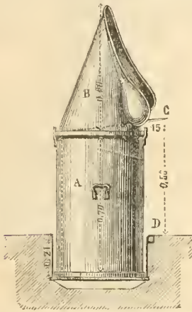
Fig. 19. — Élévation d'un urinoir mobile absorbant les urines.
