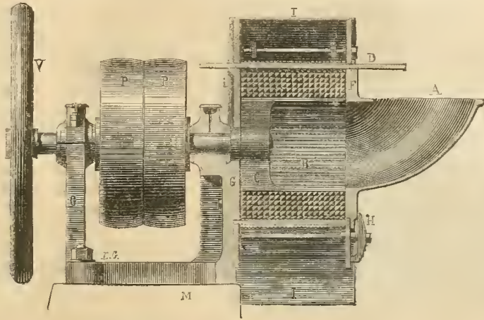
Fig. 26. — Coupe de la rape Champonnois.
