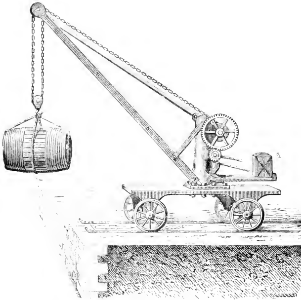
Fig. 25. — Grue roulante de MM. Mabillet.
