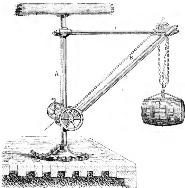
Fig. 24. — Grue tournante construite par MM. Mabille frères, à Amboise (Indre-et-Loire).
