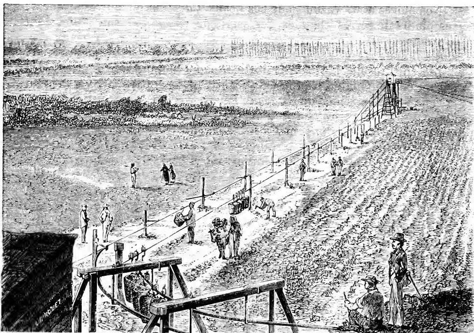
Fig. 34. — Vue d'ensemble du câble aérien automatique établi par M. Provins, à Séelowitz (Autriche).
