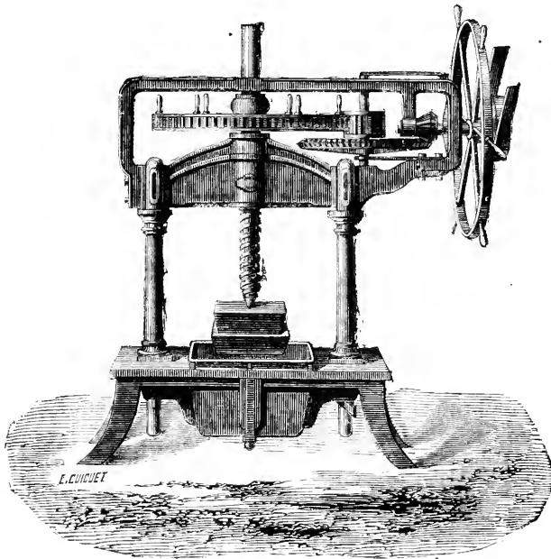
Fig. 7. — Presse à huile avec dynamomètre, à débrayage de sûreté, construite par MM. Mabilie frères, à Amboise.
