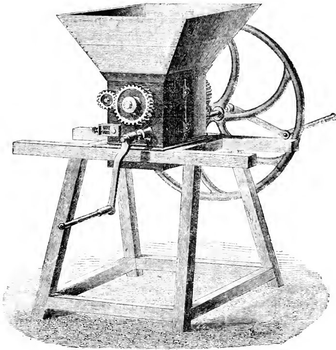
Fig. 11. — Moulin à pommes, construit par MM. Mabile frères.
