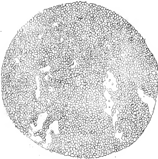
Fig. 4. — Lait vu au microscope avant le barattage.
