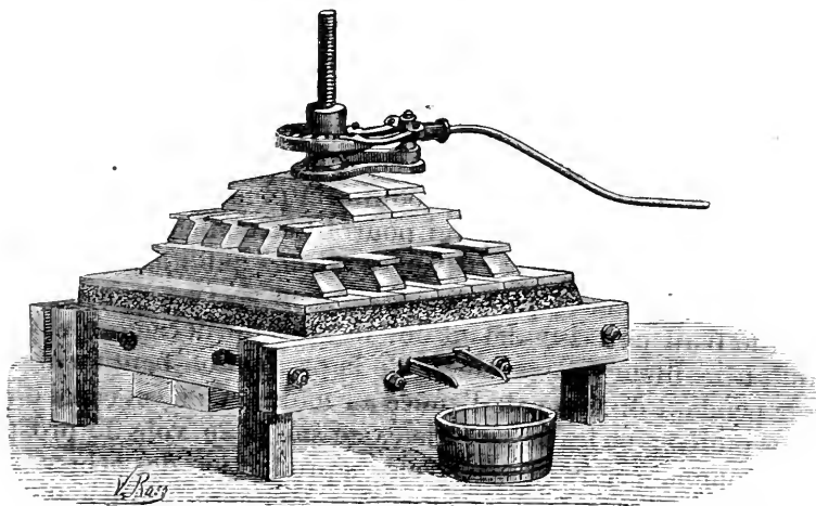
Fig. 29. — Pressoir universel Mabille avec charge carrée sans claie circulaire.
