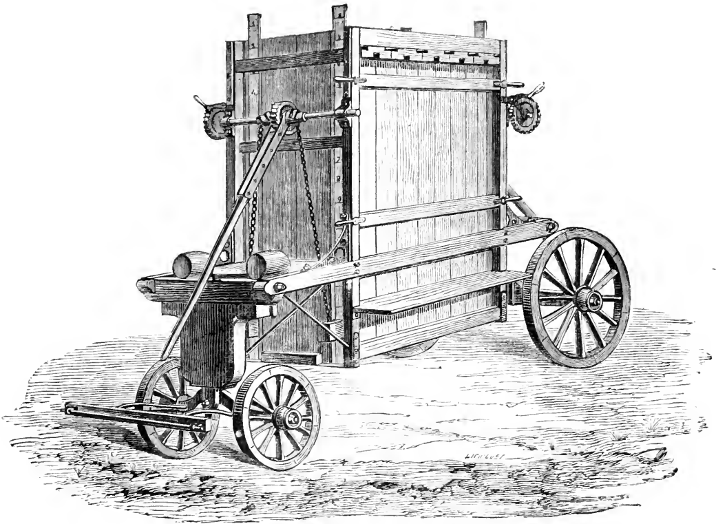
Fig. 42. — Nouvelle presse à foin inventée et construite par M. Albaret, ingénieur-constructeur à Liencourt-Rantigny (Oise).
