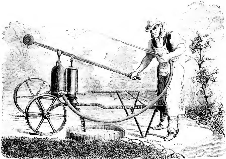
Fig. 4. — Pompe à double effet de M. Noël, à piston vertical.
