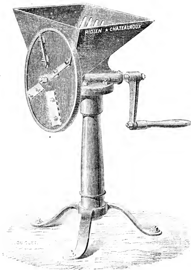
Fig. 29. — Coupe-racines à colonne de M. Hidién.
