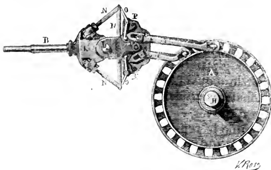
Fig. 28. — Plan du levier multiple à dynamomètre
