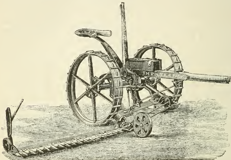
Fig. 7. — Nouvelle faucheuse système Wood.
