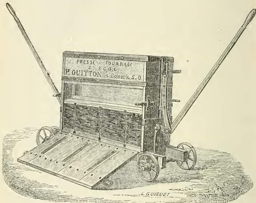
Fig. 23. — Nouvelle presse à fourrage, système Guitton.
