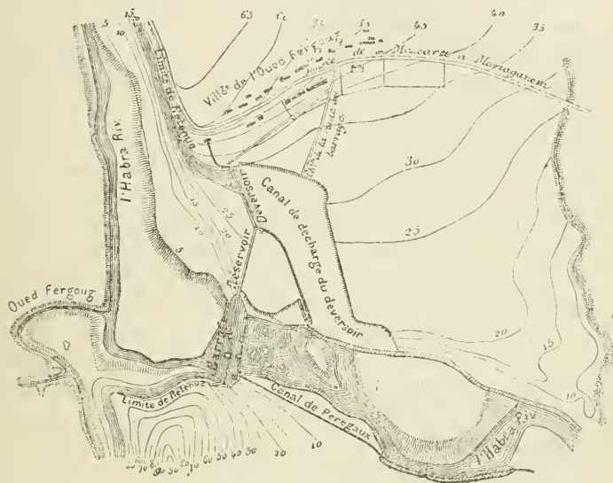
Fig. 6. — Plan du barrage de l'Habra.
