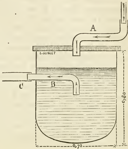
Fig. 31. — Appareil purificateur de l'eau des toits.
