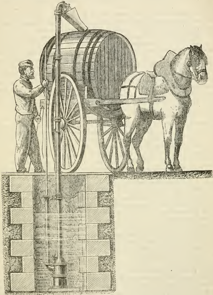
Fig. 36. — Fonctionnement de la pompe Fauler.
