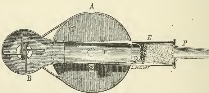
Fig. 2. — Coupe de l'enfumoir Delaplace.
