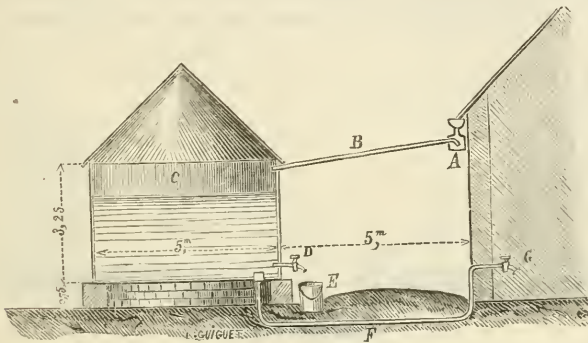
Fig. 29. — Réservoir de 60,000 litres, séparé de la grande cave par un chemin de service.
