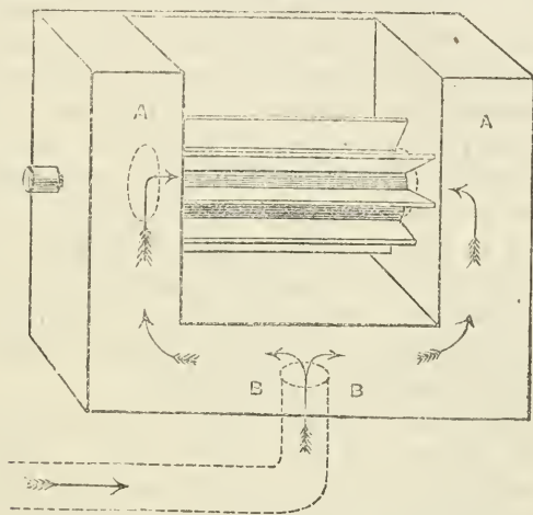
Fig. 28. — Coupe du ventilateur-aspirateur.
