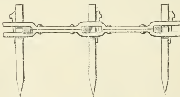
Fig. 71. — Mode d'assemblage des dents.
