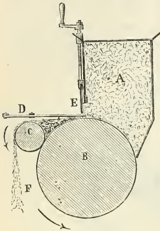
Fig. 76. — Appareil de distribution des engrais.
