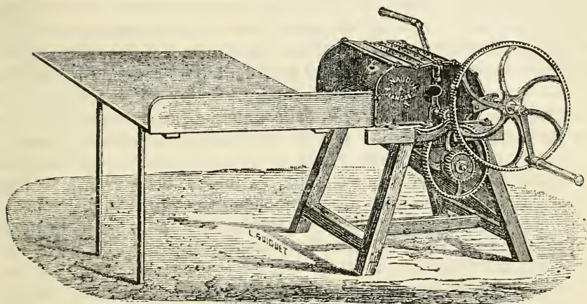
Fig. 28. — Égreneuse construite par M. Naudot.
