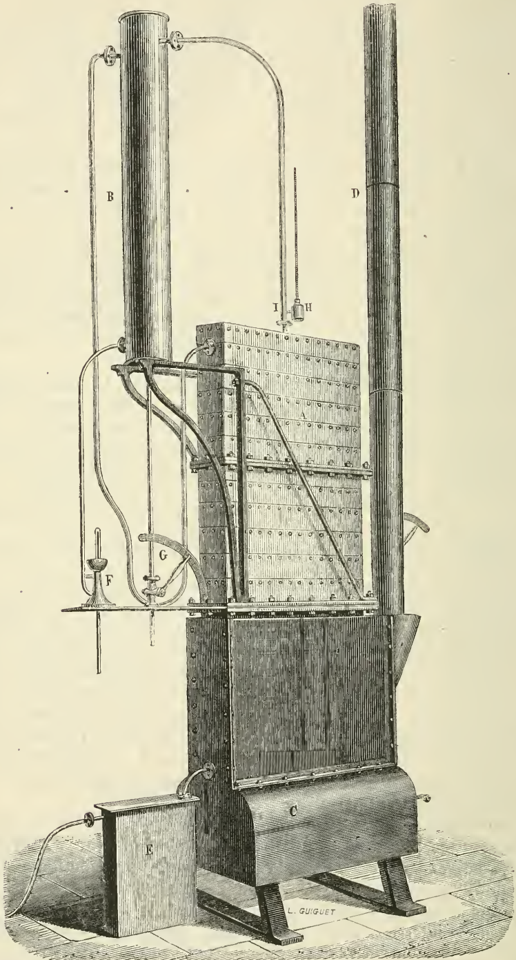
Fig. 34. — Appareil Savalle pour la fabrication continue des eaux-de-vie.
