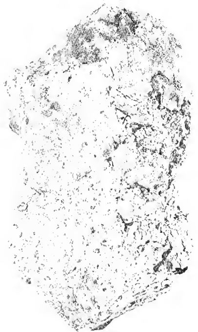
Fig. 45.—A lithoidal ceramicite. Loc.: Koiké. 16×9 cm.
