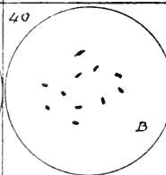
26 Scoparino alc 210
