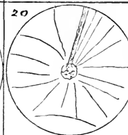
16 Strychnin chlor 55
