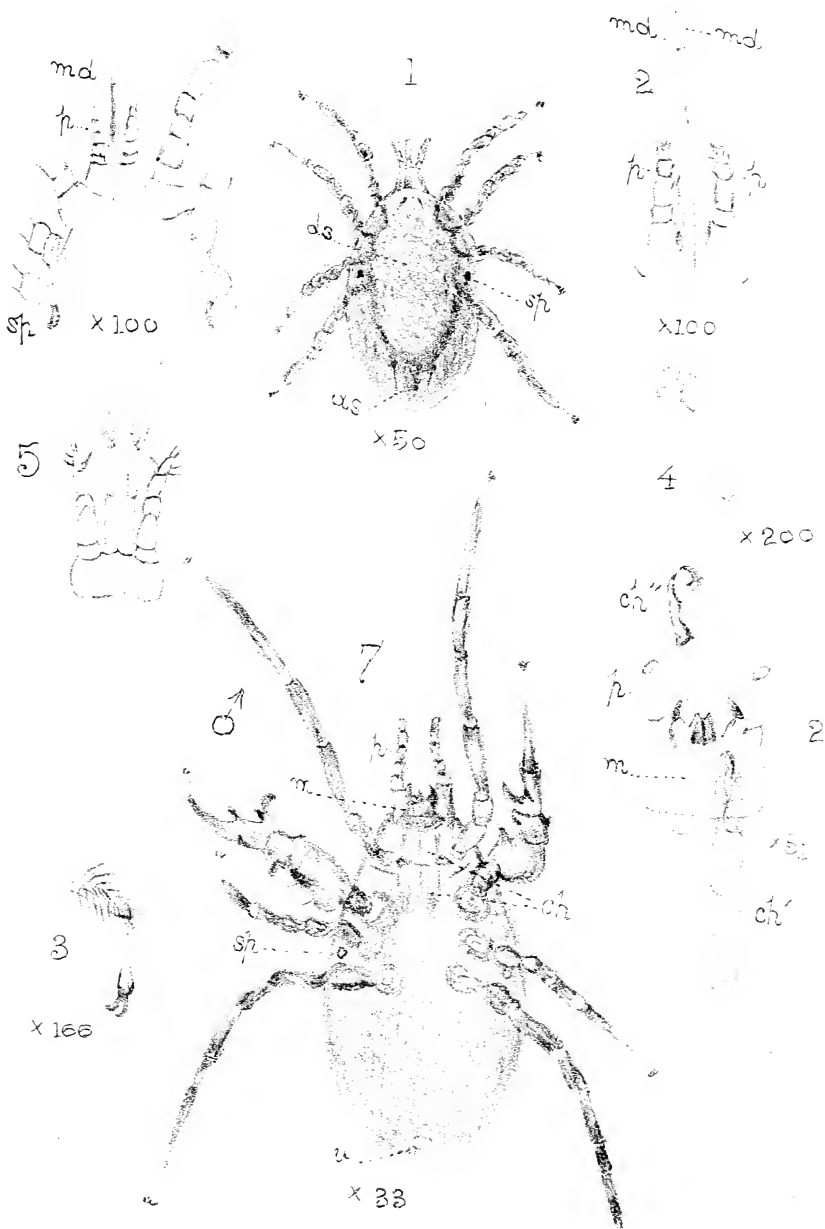
Dermanyssa.
