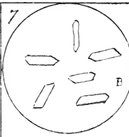
8 Narcotin alc 55
