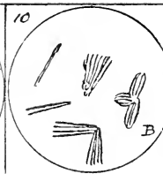
11 Papaverine alc 210
