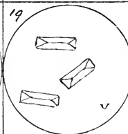
15 Atropin alc 210
