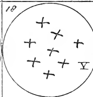
14 Amygdaline alc 210
