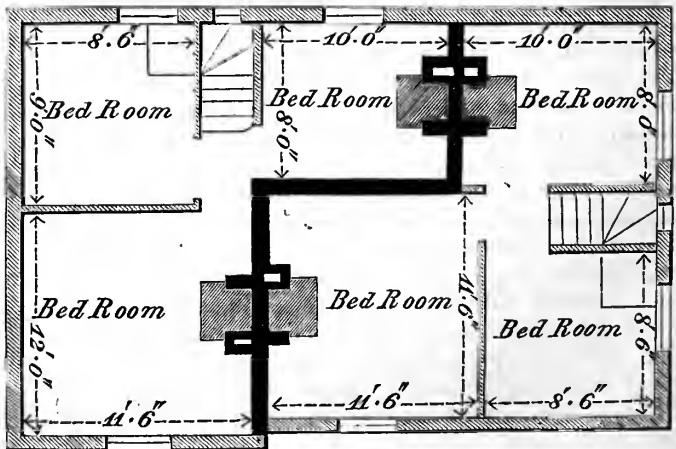
Fig. 6.—Chamber Plan.
