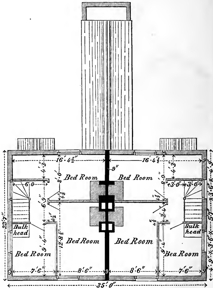
Fig. 3.—Chamber Plan.
