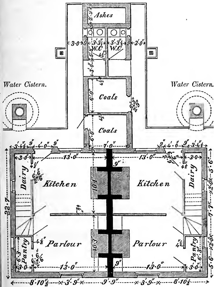
Fig. 2.—Ground Plan.
