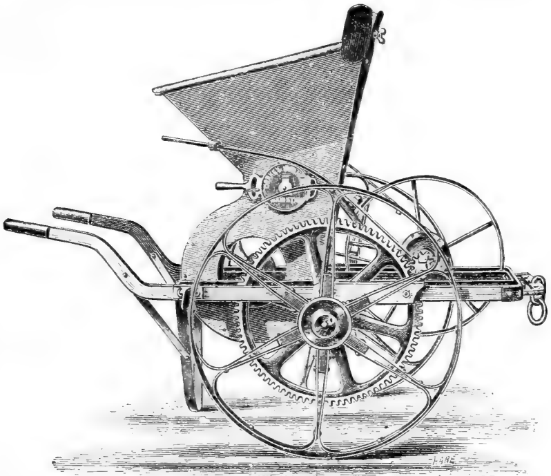
FIG. 26.—Hop sulphurator.
