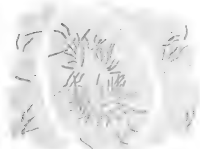
Fig. 9. HORSE. (Lung)
