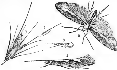
FIG. 1.—PLUTELLA CRUCIFERARUM.
