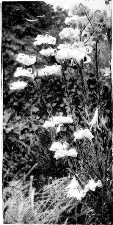
FIG. 22.—LILIIUM EXCELSUM.
