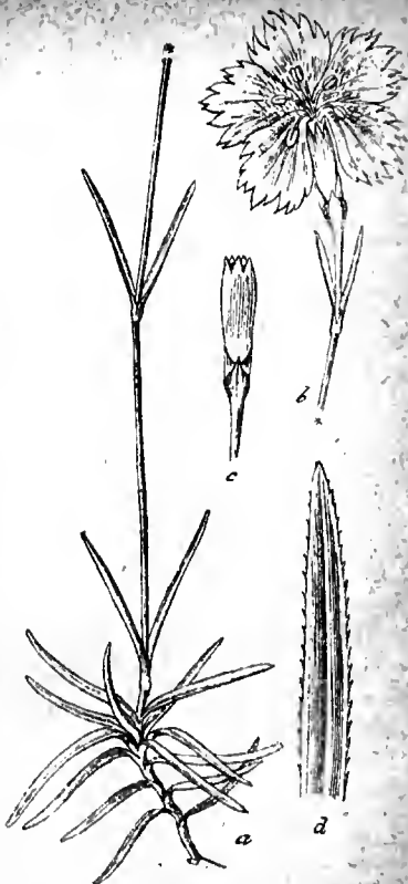
20. Pflanz-Nelke, Silene caesia . a—b) Trieb in nat. Gr.; c) Kelch in nat. Gr.; d) Blatt, vergr.
