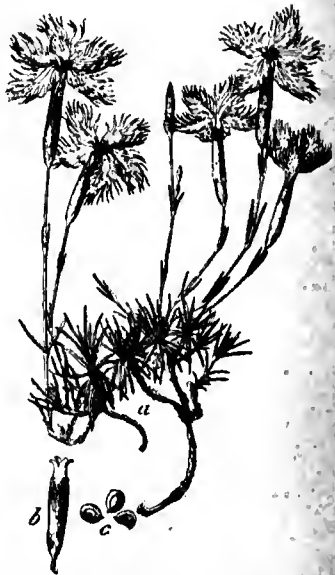
22. Sand-Nelke, Silene arenaria . a) Pflanze, verkl.; b) aufgesprungene Frucht im Kelch, verkl.; c) Samen, wenig vergr.
