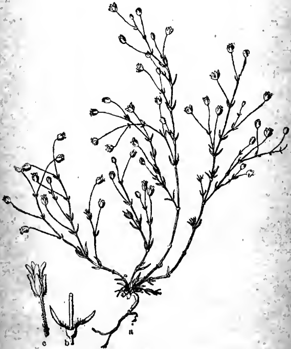
10. Niedrige Miere (grossfrüchtige Form), Alsine dubia depressa (ellipta): a) Pflanze in nat. Gr.; b) Blattpaar, vergr.; c) aufgesprungene Frucht im Kelch, vergr.
