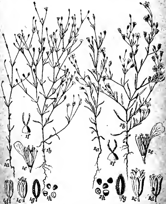
19. Maner-Nelke, Silene muralis . 1. Gewöhnliche Form. 2. Langblättrige Form mit anserandeten Kronblättern (serotina). a u. b) Pflanzen, verkl.; c) aufgesprungene Früchte im Kelch, vergr.; d) Kelche, vergr.; e) Staubgefäße und Fruchtknoten nebst einem Kronblatt, vergr.; f) Narben, vergr.; g) durchschnitene Fruchtknoten, vergr.; h) Samen nebst Durchschnitten, vergr.
