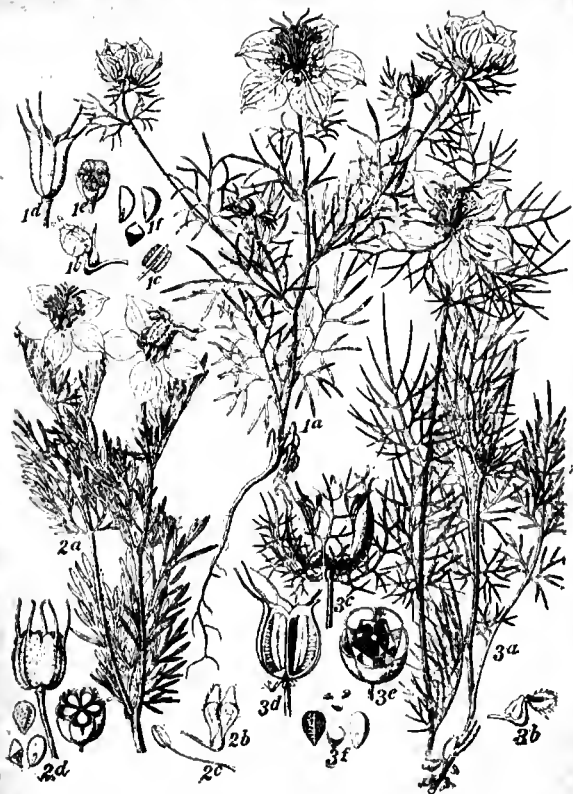
51. 1. Wilder Schwarzkümmel, Nigella arvensis . a) Pflanze, verkl.; b) Kronblatt, vergr.; c) Staubbeutel, vergr., d) Frucht, verkl.; e) durchschnittene Frucht, verkl.; f) Same nebst Durchschnitten, vergr. 2. Schwarzkümmel, Nigella sativa . a) Zweig, verkl.; b) Kronblatt, vergr.; c) Stenbgefäss in nat. Gr.; d) Frucht nebst Durchschnitten, verkl., und Same nebst Durchschnitten, vergr. 3. Jungfer im Grünen, Nigella damascena . a) Pflanze, verkl.; b) Kronblatt, vergr.; c-e) Frucht nebst Durchschnitten, verkl.; f) Samen verkl. und nebst Durchschnitten vergr.
