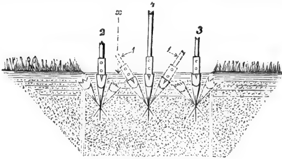
Figur 4. Verticalsechnitt eines mit dem Wühlspaten zu lockernden Platzes.
