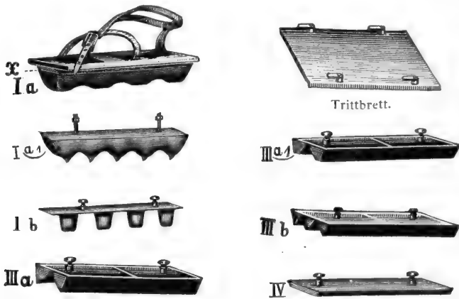
Figur 27. Rillenschuh mit Trittbrett und den anlegbaren Rillen-Formstücken.
