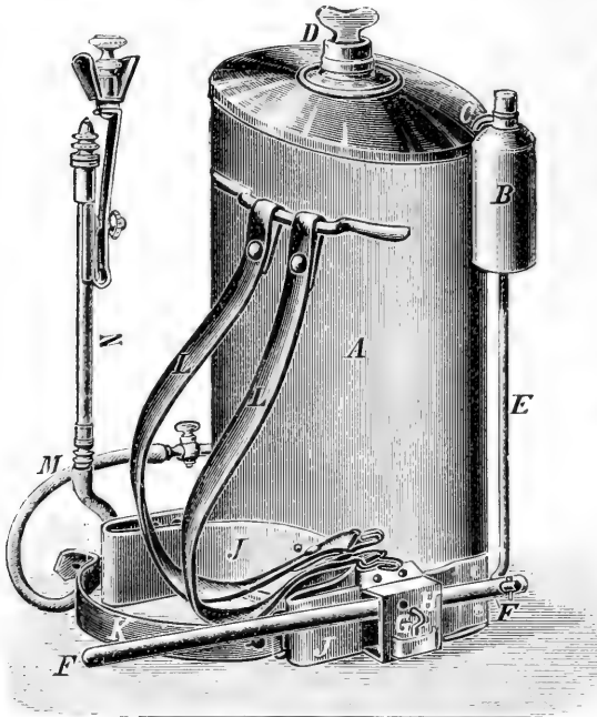
Fig. 6. Universalispritze Saxonia von Drescher in Halle.
