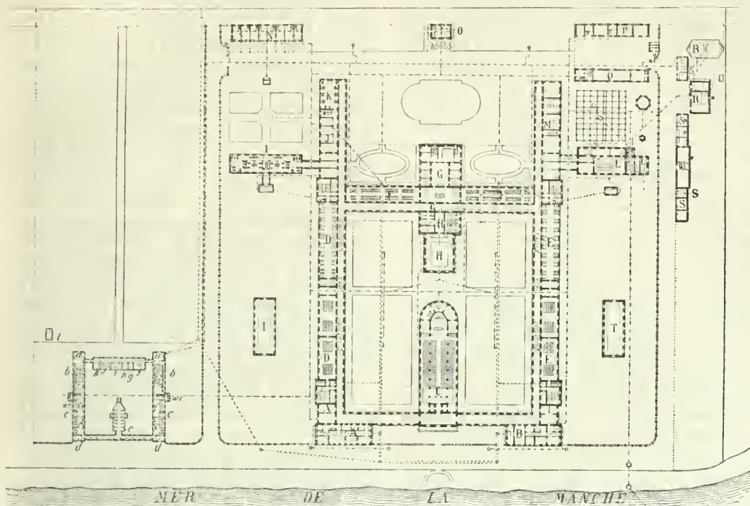
Plan de l'hôpital de Berck-sur-Mer. — A, administration, consultation ; étages, logements du personnel ; B, communauté ; C, chapelle et service des morts ; D, quartier des garçons, classes et dortoirs ; étages, dortoirs ; F, réfectoire ; étages, dortoirs ; G, cuisine et dépendances ; H, bains et piscine ; I, service d'isolement ; J, pharmacie et dépendances ; K, infirmerie ; L, buanderie et machines ; M, lingerie ; N, logements des ouvriers ; O, aumônier ; P, écuries et remises ; Q, agence et remise ; R, usine à gaz ; S, ateliers ; T, gymnases. — Petit hôpital (rez-de-chaussée) : a, entrée ; b, réfectoires ; c, dortoirs ; c', surveillantes ; d, chambres ; e, chapelle transformée en classes ; f, cuisine ; g, salle des médicaments ; h, salle de visite ; i, lingerie ; j, infirmerie ; k, surveillante ; l, photographie.
