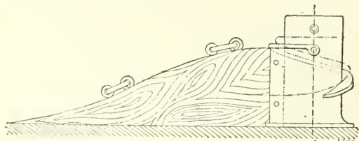
Fig. 1. — Bitte de mouillage.
