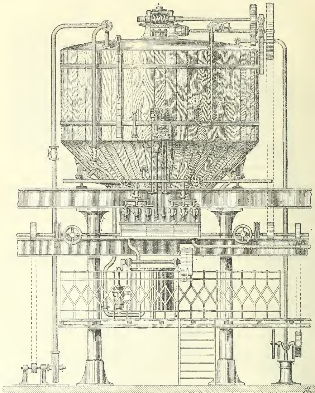
Fig. 13. — Appareil de clarification.
