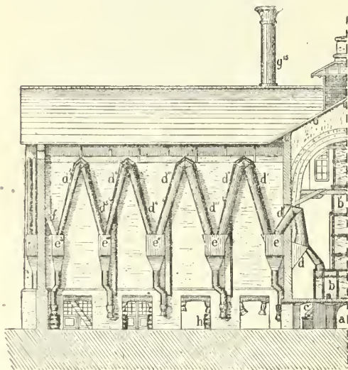
Fig. 6. — Réfrigérants retenant les premières parties de blanc de zinc entraînées. a, Cendrier; b, Fourneau distillatoire; b' b', Cheminée centrale; c e', Tuyaux conduisant l'oxyde lourd, l'air et l'oxyde léger; d, Conduit commun; d', d'', Trémies et doubles tubes; e, e', e'', Trémies closes; f, f', Trémies; g, g', g'', Chambres tapissées de toile pelucheuse; h, Barils receuillant le blanc de zinc.
