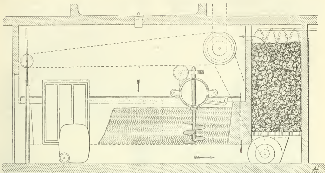
Fig. 2. — Germeoir pneumatique.
