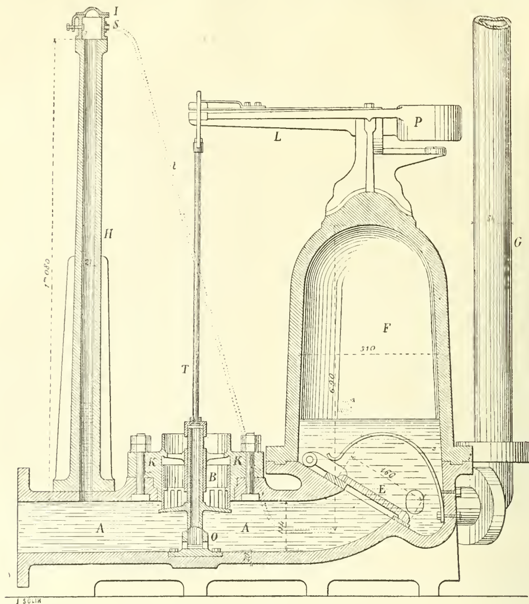
Fig. 3. — Béliet hydraulique, par M. Bolée.
