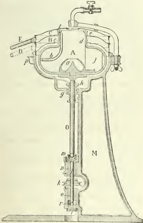
Fig. 2. — Coupe de l'écrèmeuse centrifuge Laval.
