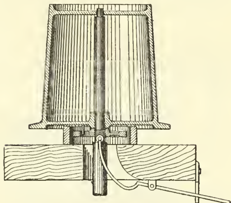
Fig. 10. — Embrayée.
