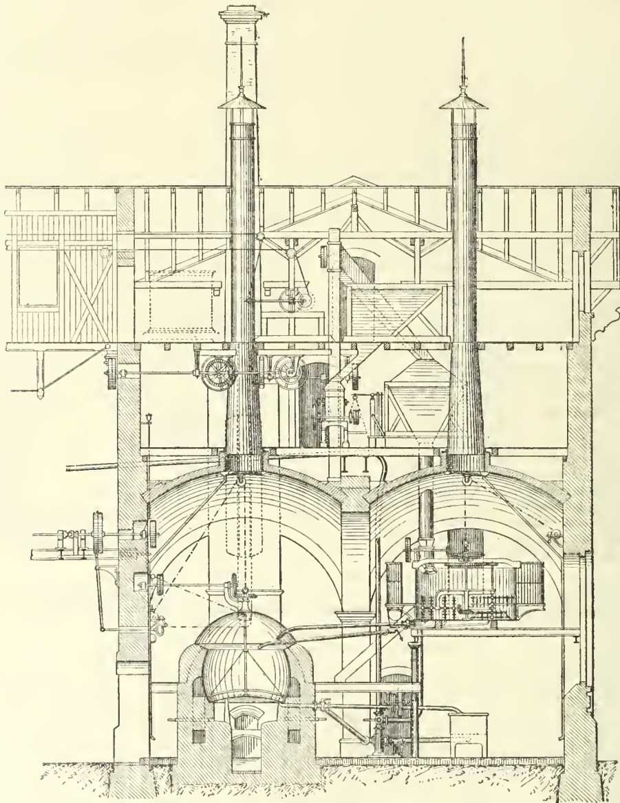
Fig. 11. — Bâtiment de cuisson.
