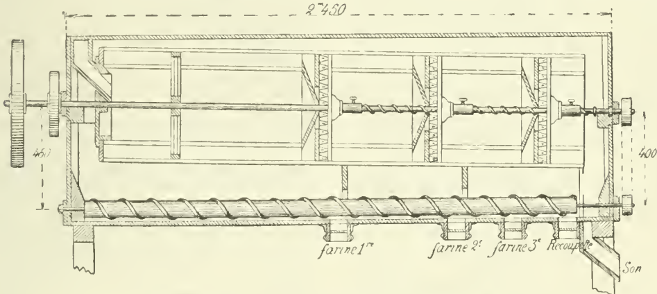
Fig. 2. — Blutoir de M. Falguière (coupe longitudinale).
