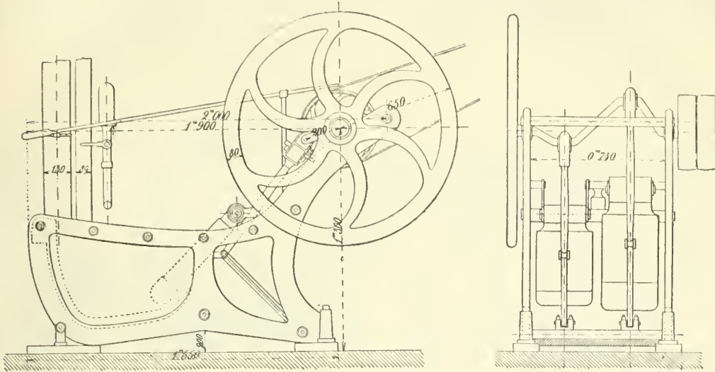
Fig. 10. — Foulon à maillets.
