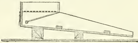
Berceau-lavoir à barrages des houilles.
