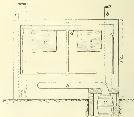
Fig. 7. — Séchoir demi-rotatif (coupe).
