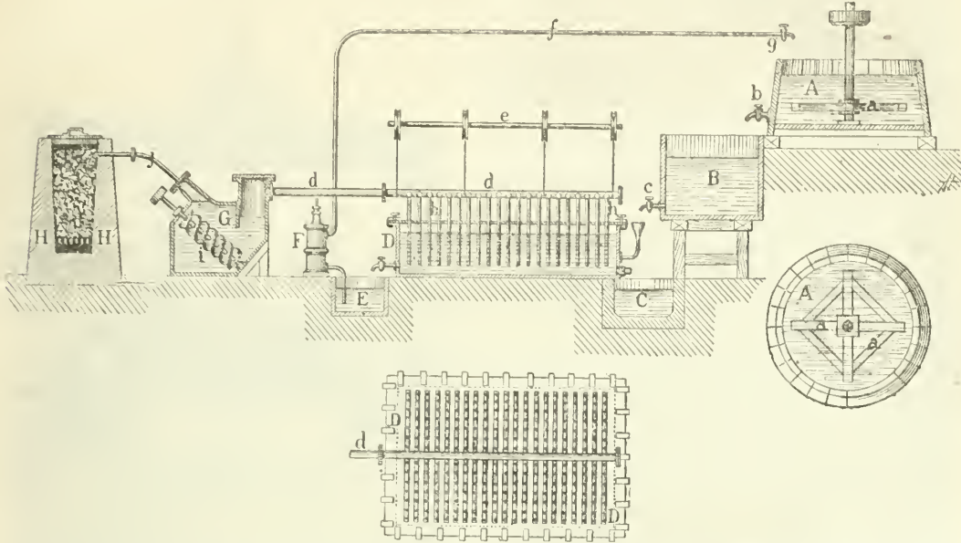
Fig. 4. — Procédé de Clichy : A, Cuve à dissolution ; B, Réservoir du liquide décanté ; C, Cuve recevant le dépôt ; D, Récipient fermé ; E, Cuve recevant le liquide clair ; F, Pompe de refoulement ; G, Cagniardelle soufflante ; H, Four à coke et à chaux ; a, Agitateur de la cuve ; b, Robinet de vidange ; c, Robinet de décantation ; d, Tuyau de refroidissement de l'acide carbonique ; e, Tringle de suspension ; f, g, Tuyau et robinet de refoulement du liquide clair ; h, Tuyau d'immersion ; i, Vis d'aspiration ; j, Tube d'aspiration de l'acide carbonique.
