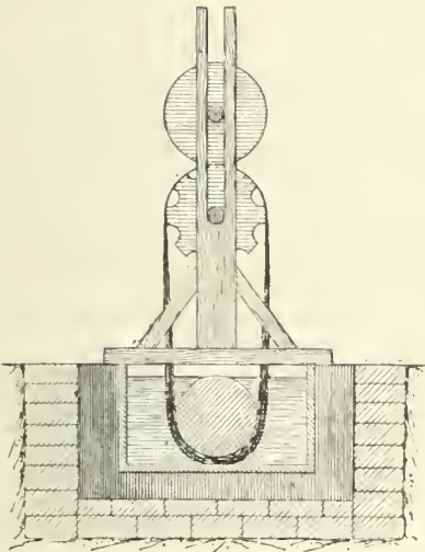
Fig. 11. — Clapot sauteur.
