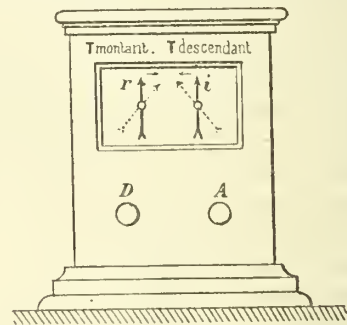
Fig. 1. — Indicateur Regnault (réseau de l'Ouest).
