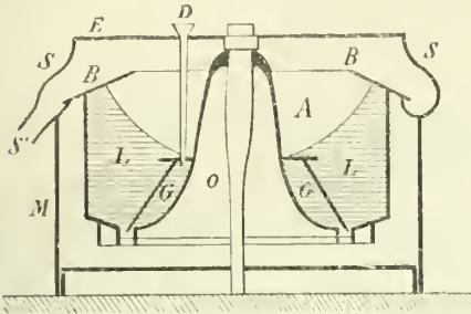
Fig. 1. — Ecrèmeuse centrifuge Lefeldt. — A, Récipient en fer blanc dans lequel on introduit le lait par le tube D; O, Axe sur lequel est fixé le récipient A et auquel on communique un mouvement de rotation très rapide; G, Cloison qui descend vers le fond du tambour, tout en laissant un petit espace libre; E, Couverte fixe; M, Manchon en tôle qui enveloppe le récipient A et qui porte à son bord supérieur une rigole S avec conduite de sortie en S'.
