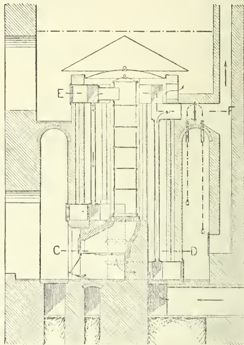
Fig. 4. — Touraille (coupe du calorifère).
