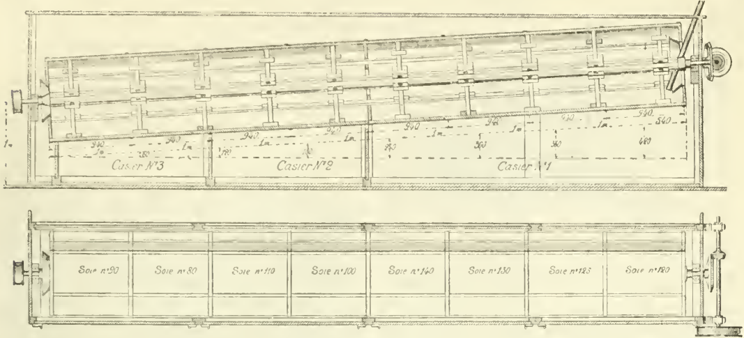
Fig. 1. — Bluterie à farine.
