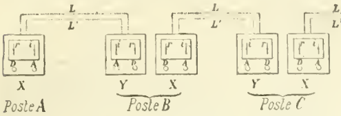
Fig. 2. — Ensemble de la disposition des indicateurs (réseau de l'Ouest).
