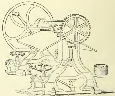
Fig. 11. — Calandre chauffée au fer ou à la vapeur, à moteur ou à bras.
