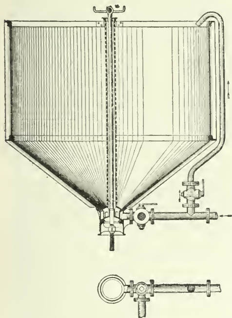
Fig. 1. — Cuve-mouilloir.
