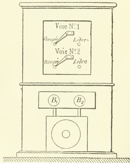
Fig. 4. — Appareil Tyer (réseau de Lyon).
