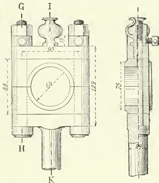
Fig. 4. — Élévation et coupe par GH et IK.
