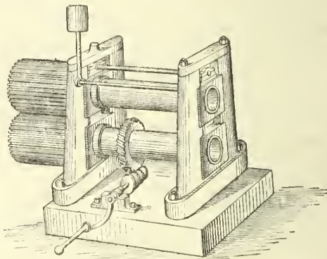
Fig. 12. — Machine à tuyauter.
