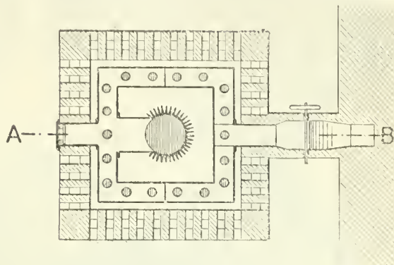
Fig. 6. — Plan du calorifère.
