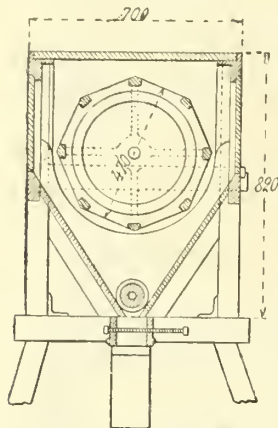
Fig. 2 bis. — Blutoir de M. Falguière (coupe transversale).
