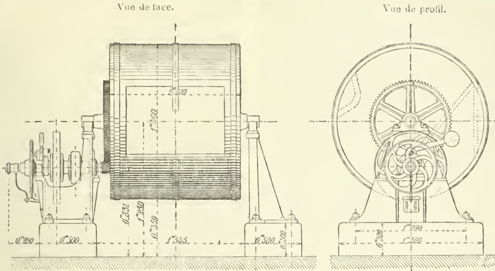
Fig. 14. — Machine à laver à spirale.
