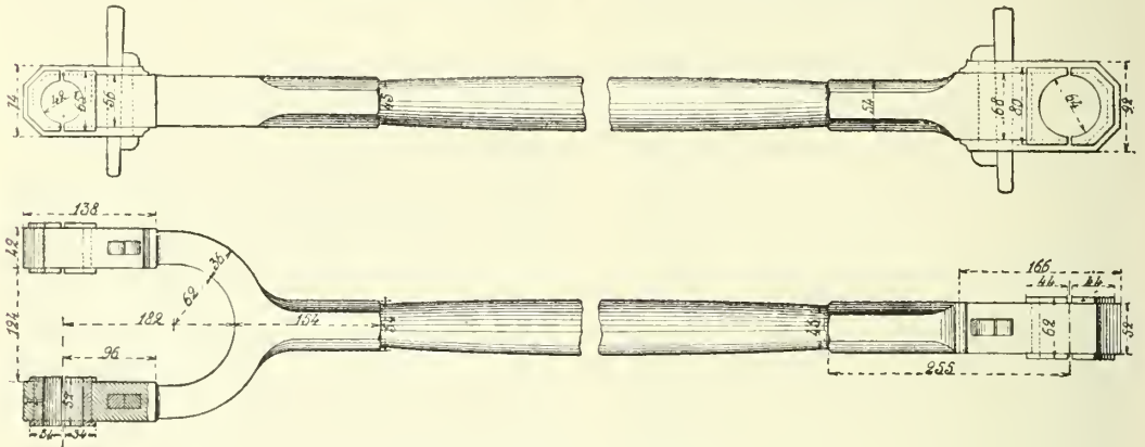
Fig. 1. — Bielle en fer forgé.
