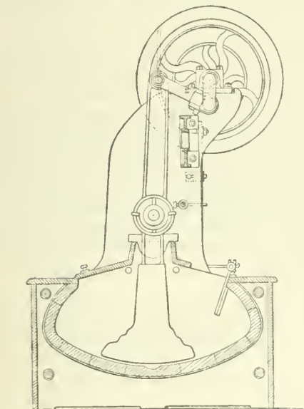
Fig. 4. — Coupe.
