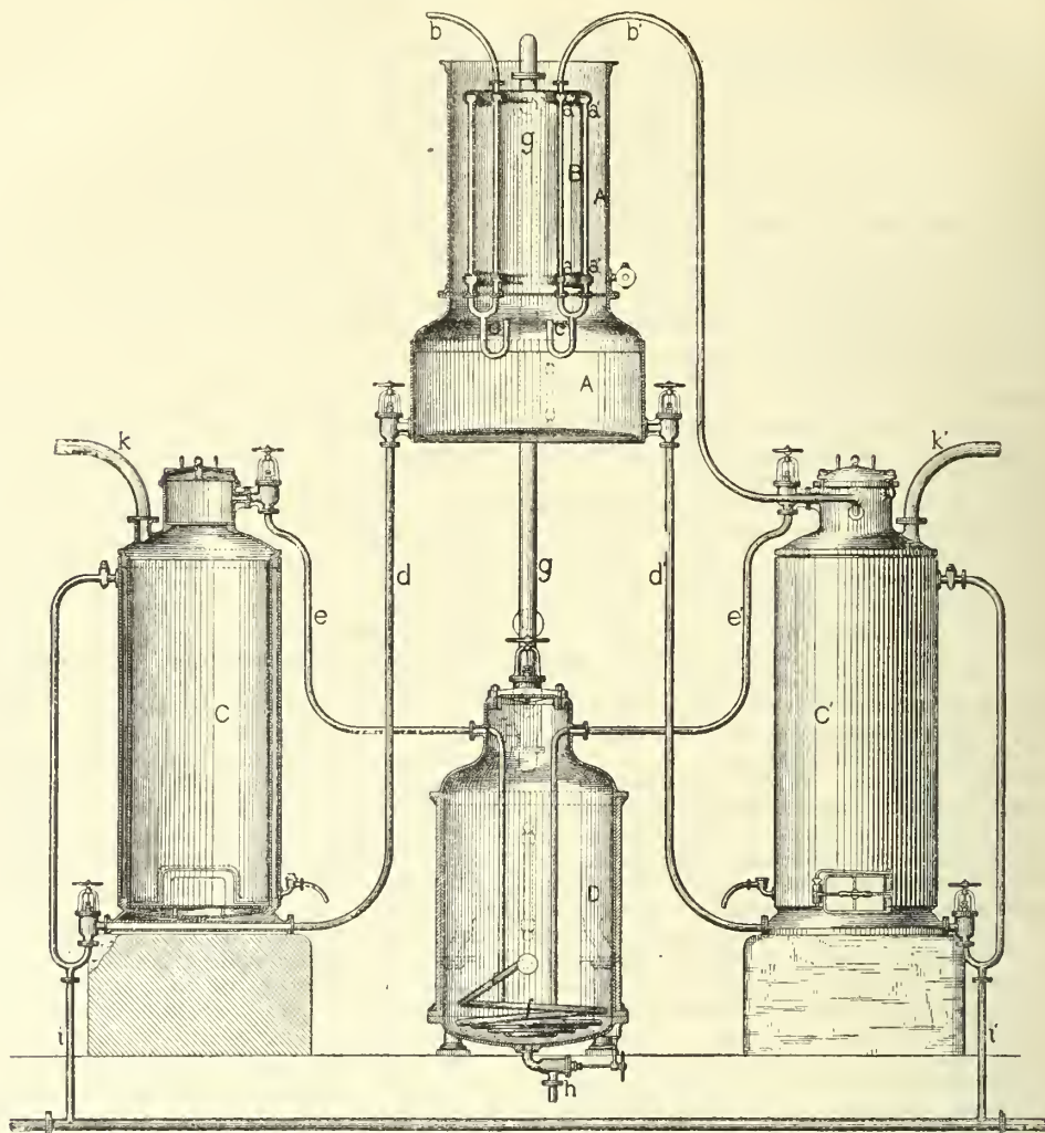
Fig. 1. — Appareil Moussu pour l'extraction des bitumes.
