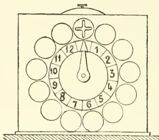
Fig. 6. — Indicateur Joussetin (réseau de Lyon).
