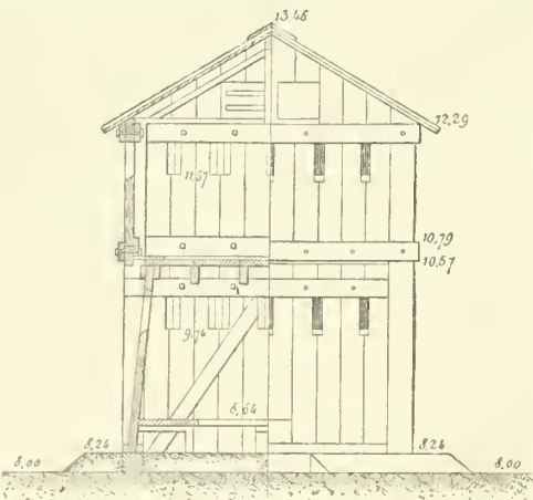
Fig. 2. — Coupe et élévation d'un blockhaus à étage. ]
