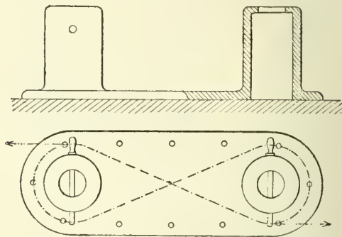
Fig. 2. — Bittes de remorque.
