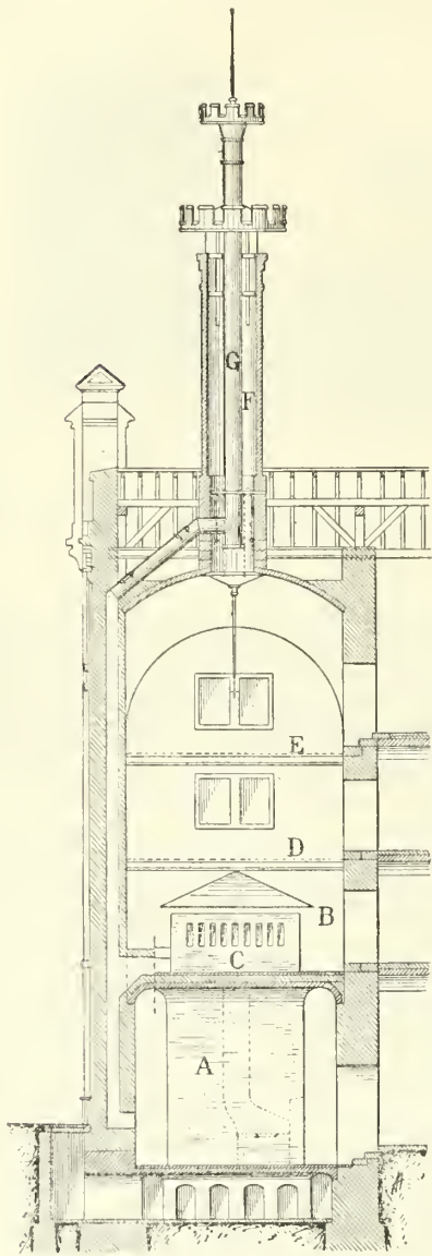
Fig. 3. — Touraille. A, calorifère; B, chambre à air chaud; C, ouverture pour la sortie de l'air chaud; D, E, claies formant les cloisons des compartiments de la touraille; F, cheminée destinée à enlever la vapeur d'eau; G, cheminée du calorifère.
