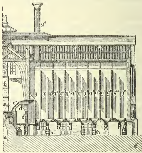
Fig. 7. — Chambre tapissée de toile pour retenir les dernières parties de blanc de zinc entraînées. c e', Tuyaux conduisant l'oxyde lourd, l'air et l'oxyde léger; d, Conduit commun; d', d'', Trémies et doubles tubes; e, e', e'', Trémies closes; f, f', Trémies; g, g', g'', Chambres tapissées de toile pelucheuse; h, Barils receuillant le blanc de zinc.
