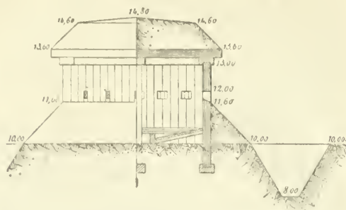
Fig. 1. — Coupe et élévation d'un blockhaus ordinaire.
