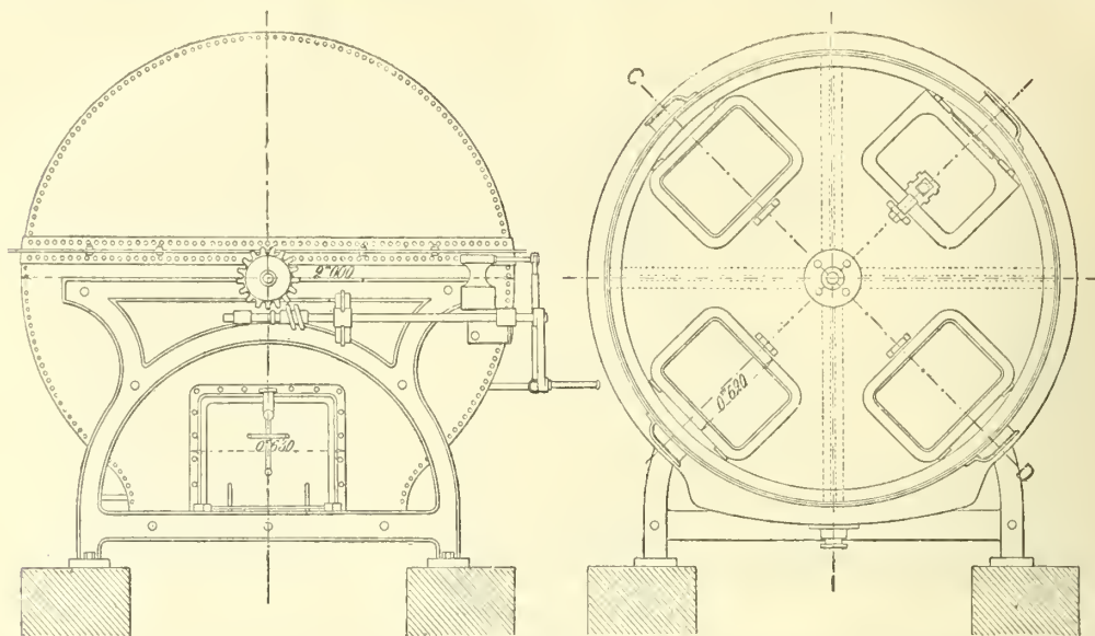
Fig. 13. — Roue américaine.
