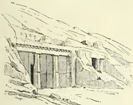
Tombeau d'Améni-Aménemhâ.
