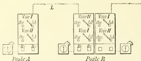
Fig. 5. — Ensemble des appareils de deux postes Tyer consécutifs (réseau de Lyon).
