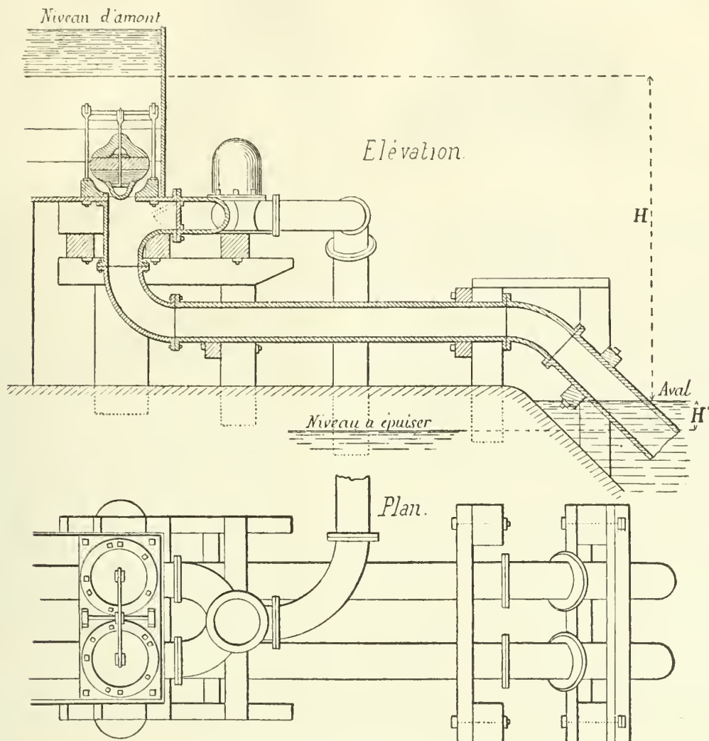
Fig. 4. — Bélier d'épuisement, par M. Leblanc.
