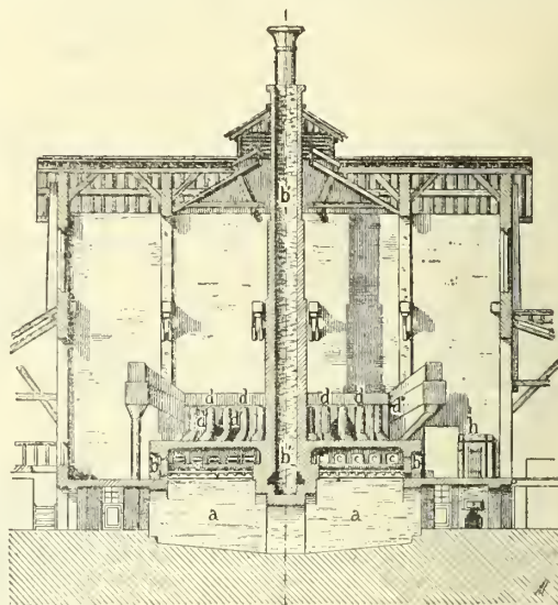
Fig. 5. — Four silésien pour la fabrication du blanc de zinc: a, Cendrier; b b, Fourneaux distillatoires; b' b', Cheminée centrale; c, Tuyaux conduisant l'oxyde lourd, l'air et l'oxyde léger; d, Conduit commun; d', Trémies et doubles tubes; h, Baril receuillant le blanc de zinc.
