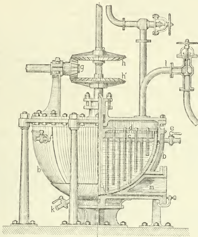
Fig. 2. — Broyeuse pour bleu de diphenylamine : a, cuve plongeant dans le double fond b chauffé à la vapeur ; c, agitateur à ailettes montées sur le fond de la cuve a ; d, agitateur à ailettes montées sur un plateau ; les deux agitateurs étant mus en sens inverse par les engrenages g, h, h' ; e et f, robinets d'entrée et de sortie de vapeur ; k, robinet d'introduction de vapeur dans l'appareil ; l, tuyaux de cohobation et de distillation ; m, trou de coulee.
