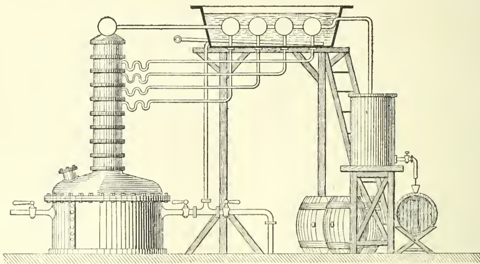
Fig. 2. — Appareil Coupier.
