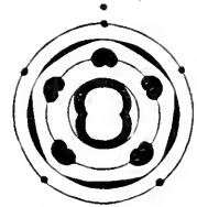
Fig. 300. Diagramm der Compositenblüte.
