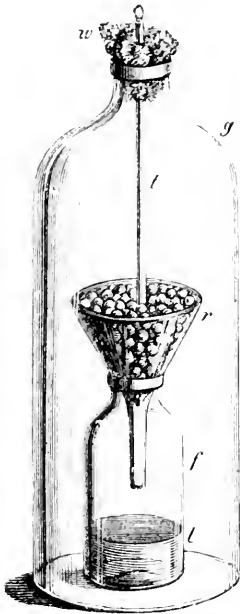
Fig. 80. Apparat zur Beobachtung der Selbsterwärmung kleiner, sich öffnender Blüten oder keimender Samen. Dieselben werden auf den Trichter r möglichst dicht zusammengehäuft und dieser in ein unten Kallilunge ( l ) enthaltendes Gefäß ( f ) gesteckt. Dieselbe absorbiert die bei der Athmung gebildete Kohlensäure. Das Ganze wird mit einer Glocke ( g ) bedeckt, durch deren mit Baumwolle locker verstopften Hals ein feines Thermometer geführt wird, dessen Kugel zwischen den Objekten steckt. Die Temperatur wird in diesem Apparat höher sein als in einem zweiten ebensolchen, zum Vergleich aufgestellten, in dem die Pflanzentheile durch Papierstücke u. dgl. ersetzt sind (nach Sachs).
