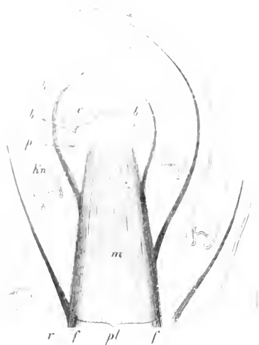
Fig. 1. Schematischer Längsschnitt durch eine Stengelspitze, bb die Blätter, welche nach oben zu immer jünger, am Vegetationspunkte sich bilden, kn deren Achselknospen.
