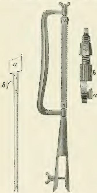
Fig. 115. Stoßeisenstange.
