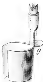
Fig. 112. Heyerische Hohlbohrer.
