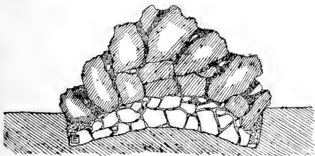
Fig. 5. — Construction (coupe) d'une rocaïlle en terrain plat.
