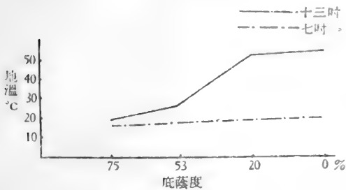
图5 底蔭度与地温关系
