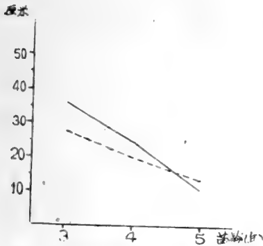
图3 单位面积密度与兴安落叶松幼树年高生长的关系(0.3 郁闭度区)
