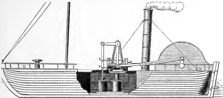
MACHINERY OF THE 'CHARLOTTE DUNDAS.'
