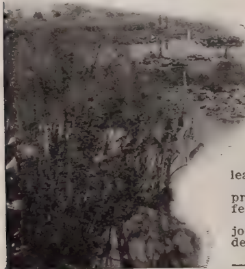
Cyperus Papyrus.
