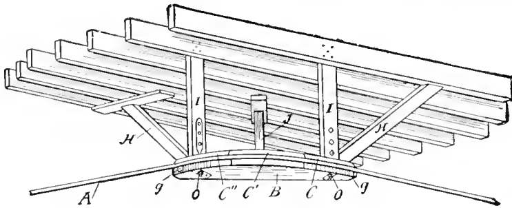
Fig. 797. (Tense.) Patented Mar. 31, 1908
