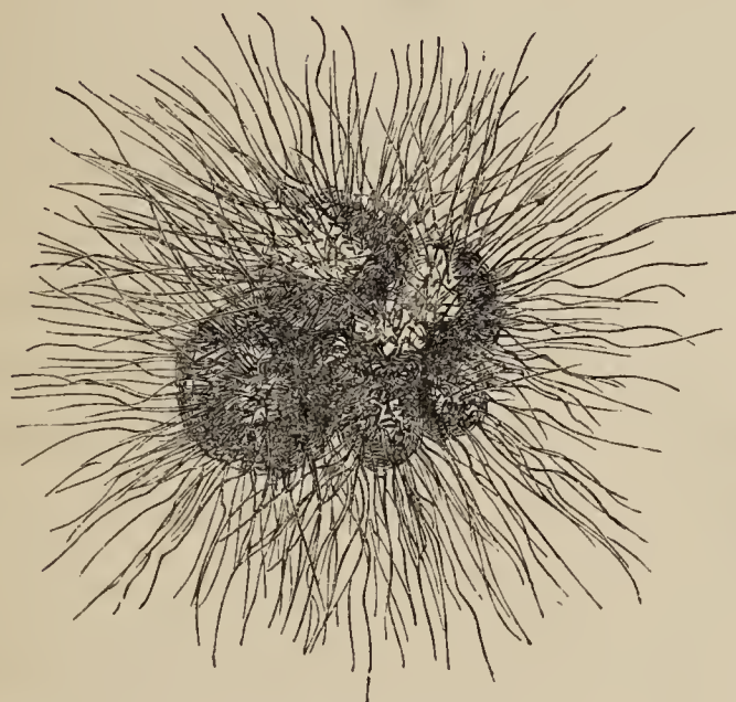
GLOBIGERINA.
