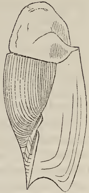
Fig. 20. Cymba .*
