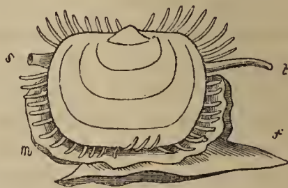
Fig. 215. Lepton .
