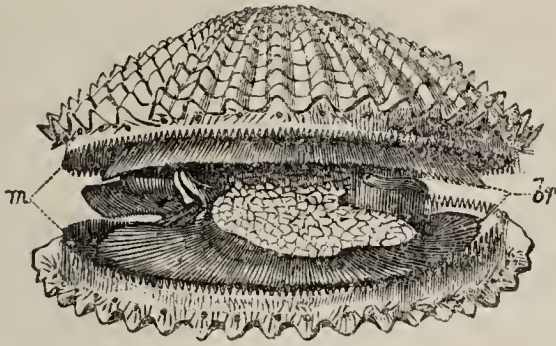
Fig. 10. Pecten varius .*
