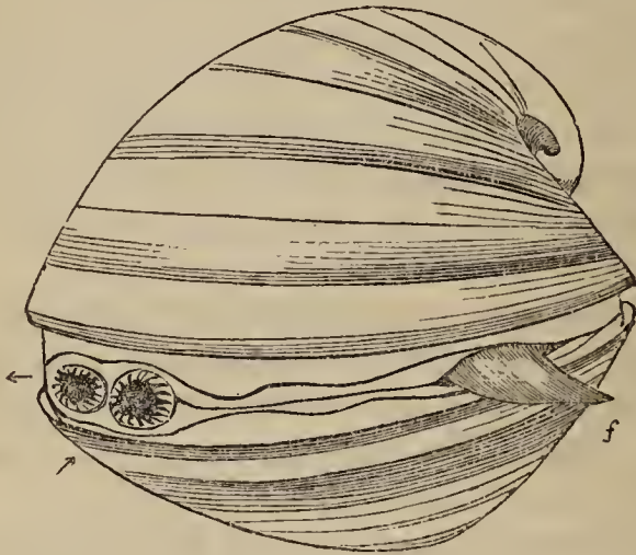
Fig. 217. Isocardia cor .
