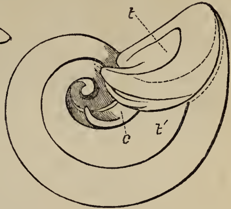
Fig. 191. Requiensia , \frac{1}{2} .
