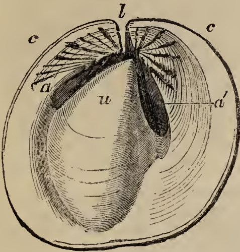
Fig. 205. Upper view.
