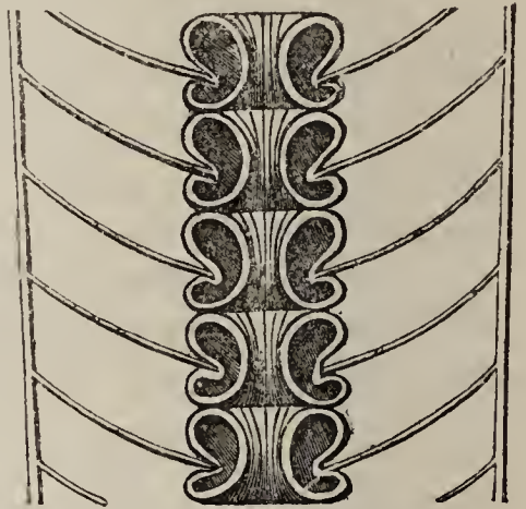
Fig. 48. Ormoceras .
