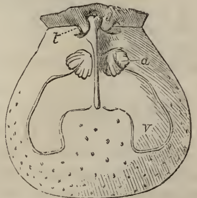
Fig. 155. S. Morrisii.
