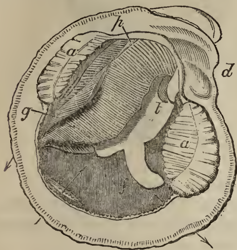
Fig. 184. Right Side.
