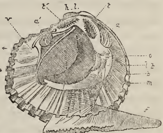
Fig. 18. Trigonina pectinata .*
