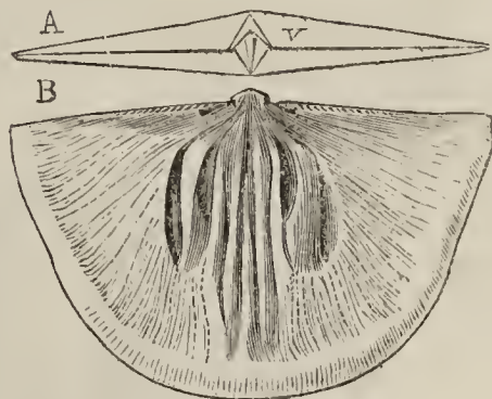
Fig. 150. Leptæna . \frac{2}{1}
