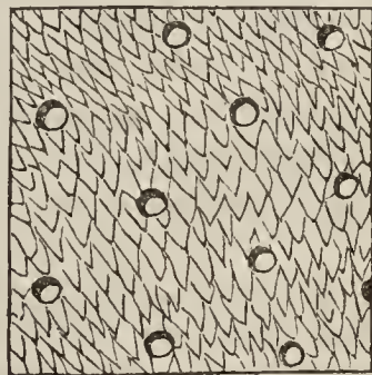
Fig. 110. Terebratula .
