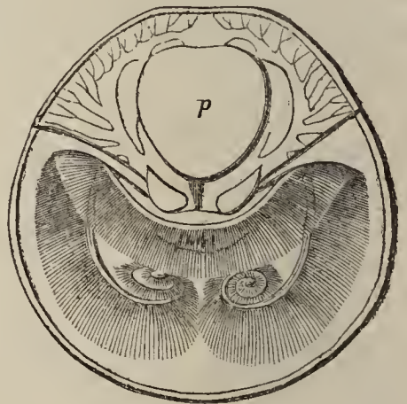
Fig. 160. Discina .‡
