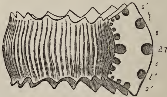
Fig. 56. Ammonites coronatus .*
