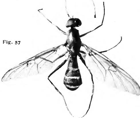
Fig. 55. Chrysochloa . Fig. 56. Rhaphiocera . Fig. 57. Plecticus .
