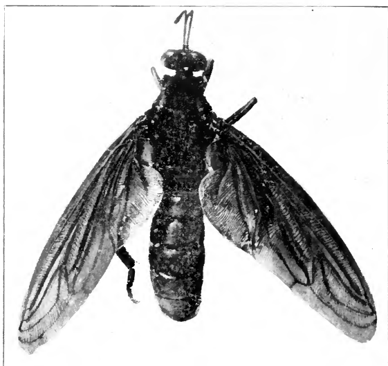
Fig. 1. Mydas , species indet. Life size. (Brazil.)
