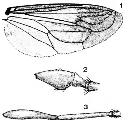
Fig. 72. Mydaiidæ. 1, Dolichogaster , wing; 2, Dolichogaster , antenna; 3, Mydas , antenna.
