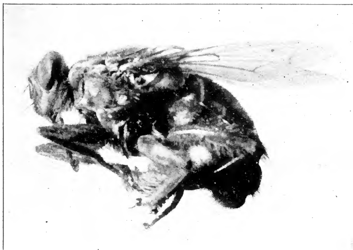
Fig. 143. Peckia praeceps , enlarged.
