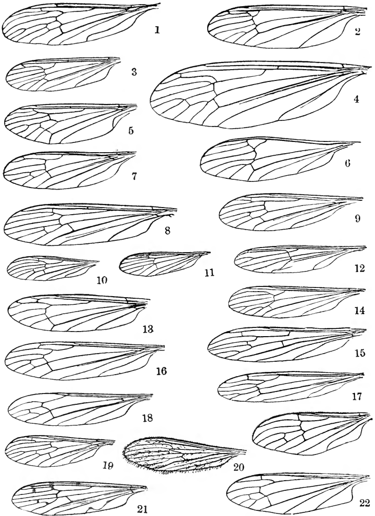
Fig. 25. Tipulidæ. 1, Limophila luteipennis ; 2, Dicranota rivularis ; 3, Plectromyia modesta ; 4, Amalopsis calcar ; 5, Trichocera bimacula ; 6, Cryptolabis paradoxa ; 7, Goniomyia sulphurella ; 8,
