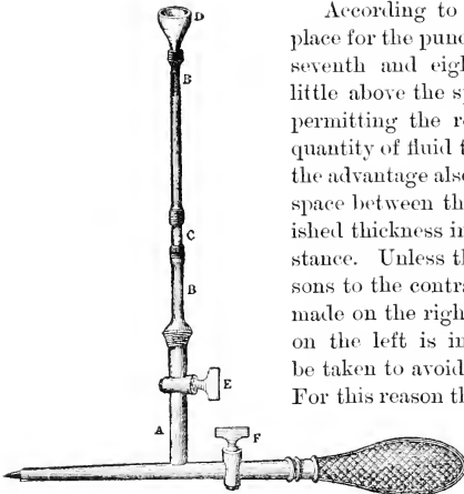
FIG. 434.—Trocar paracento-injecteur de Reul.
