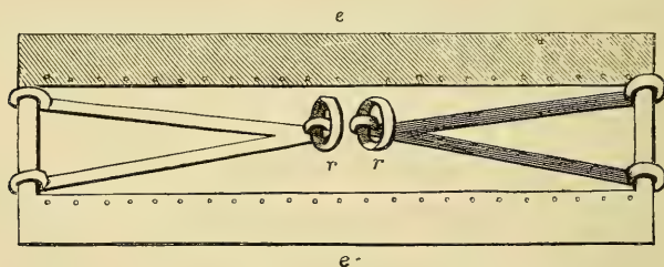
Fig. 53. — Plan du cadre de la monture d'une drague, réduit à 1/8.
