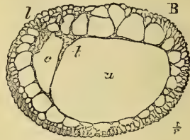
Fig. 248. — Valve spirale.
