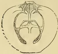
Fig. 151. — Terebratella .
