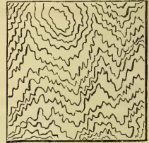
Fig. 25. — Perle 1 .
