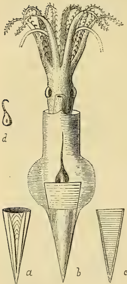
Fig. 40. — Belemnoteuthis 1 .
