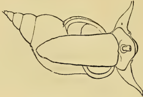
Fig. 128. — L. stagnalis .
