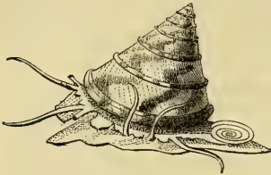
Fig. 28. — Trochus ziziphinus 1 .
