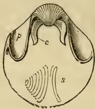
Fig. 175. — Uncites gryphus .
