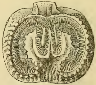
Fig. 164. — Th. Mediterraneum . 4/1 4 .
