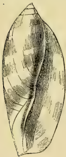
Fig. 27. — Jeune Porcelaine 2 .
