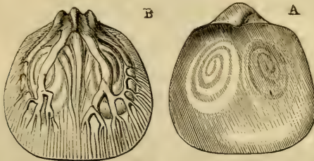
Fig. 186. — Productus? Leonhardi , 2/1 1 .
