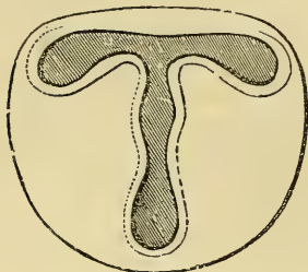
Fig. 47. — Gomphoceras 1 .
