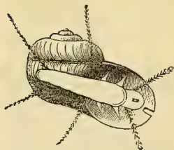
Fig. 116. — Scissurella , 8/1.
