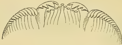
Fig 118. — Fissurella . (Wilton.)
