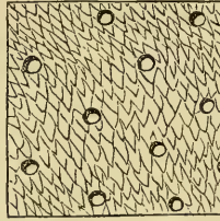
Fig. 22. — Terebratula .
