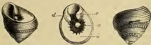
Fig. 283. — Ditremaria quinquécincta .
