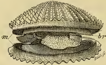
Fig. 10. — Pecten varius 2 .
