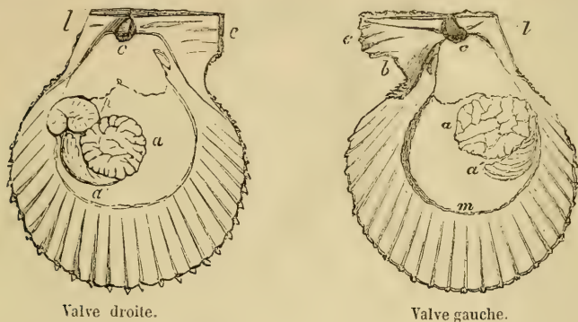
Fig. 210. — Pecten varius .
