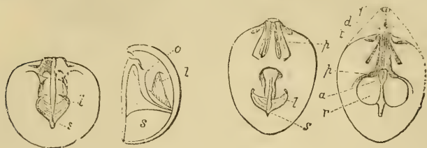
Fig. 153. — M. pumila , 2/1.
