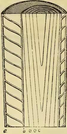
Fig. 57.— Endoceras 1 .
