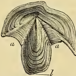
Fig. 225. — Biradiolites , \frac{5}{8} .
