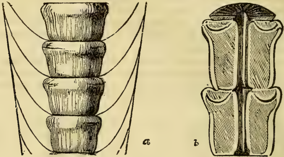
Fig. 56. — Huronia vertebralis 1 .
