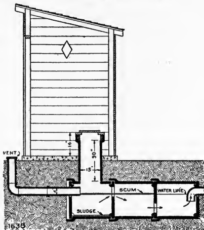
FIG. 81-a. Septic tank.
