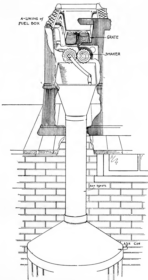
FIG. 3. Ash chute.
