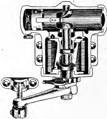
FIG. 128. Check valve.
