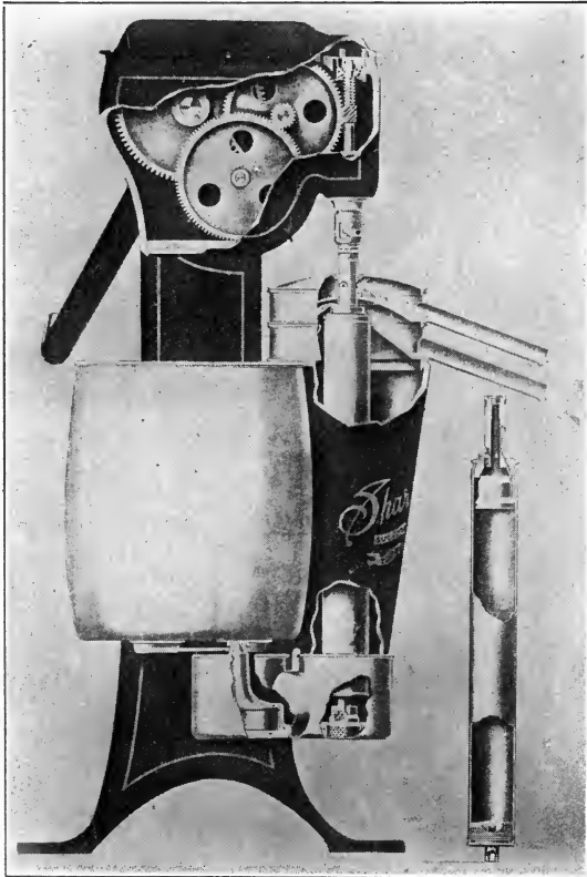
FIG. 124. Cream separator.
