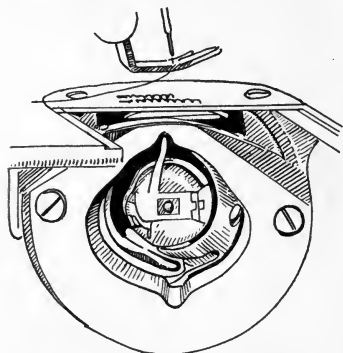
FIG. 136. Spool bobbin.
