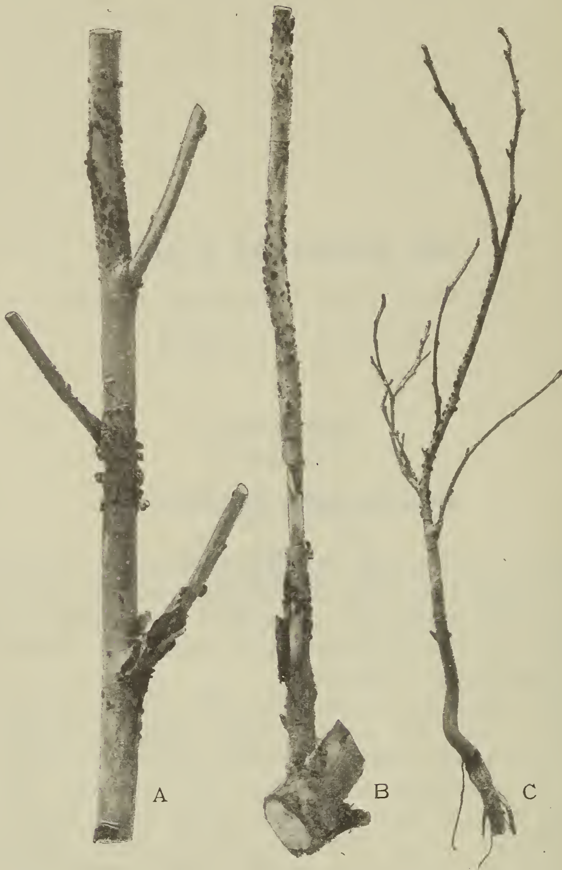
Fig. 1. A—B. Unga almgrenar, svårt angripna af grenbrand; C. En ung planta, alldeles död af sjukdomen. \frac{3}{5} 1905.
