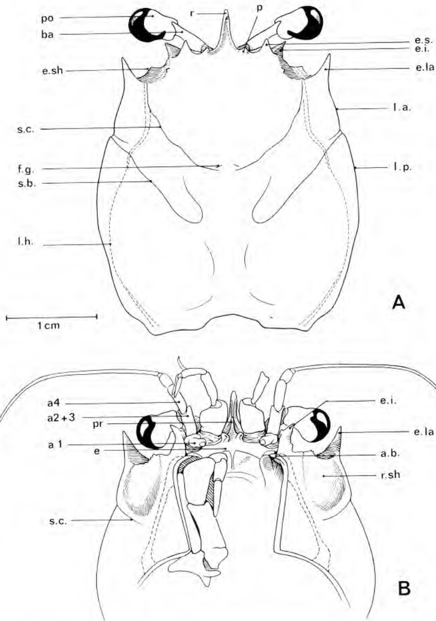
FIG. 19. — Représentation schématique de la face dorsale (A) et de la face ventrale (B) antérieures dans le genre Paromolopsis Wood-Mason : P. boasi Wood-Mason, ♂ 36 x 30 mm, Madagascar, st. 25 (MNHN-B 17105). (Pilosité non représentée). a1, article urinaire de l'antenne ; a2+3, article basal antennaire ; a4, article antennaire 4 ; a. b., auvent buccal ; e, épistome ; e. i., épine infra-orbitaire ; e. la, dent ou épine latéro-antérieure ; e. s., épine supra-orbitaire ; e. sh, épine sous-hépatique ; f. g., fossettes gastriques ; l. a., bord latéro-antérieur ; l. h., ligne homolienne ; l. p., bord latéro-postérieur ; p, épine pseudo-rostrale ; po, podophtalmite ; pr, proépistome ; r, rostre ; r. sh, région sous-hépatique ; s. b., sillon branchio-cardiaque ; s. c., sillon cervical ou gastrique.
