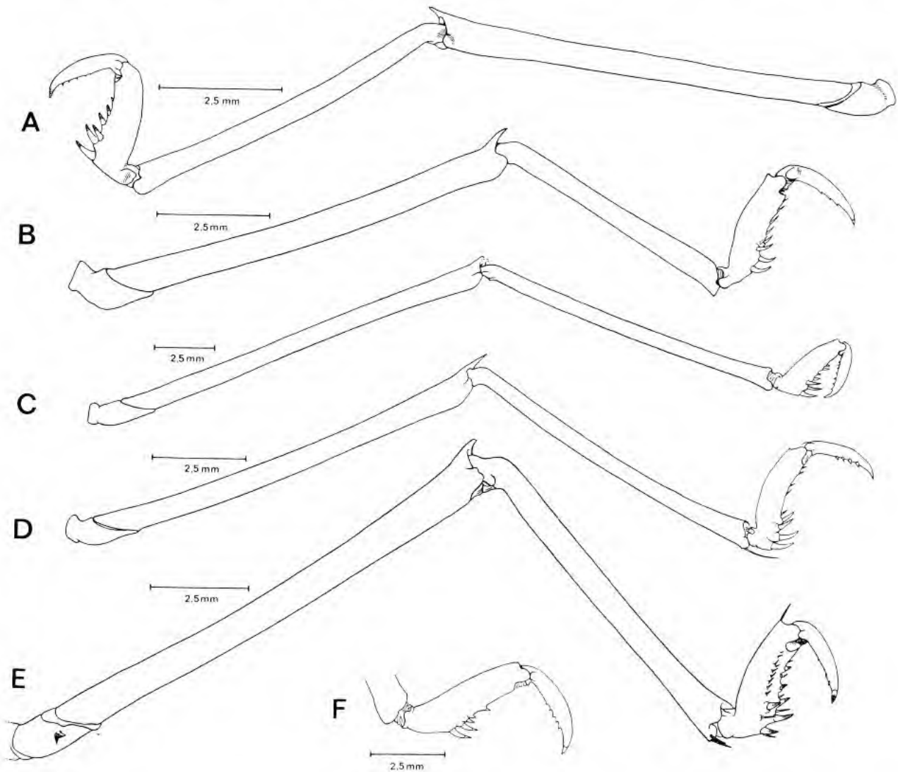
FIG. 43 A-E. — P5 : A , Latreillopsis bispinosa Henderson forme trispinosa , ♂ 9 x 6,4 mm, Philippines, MUSORSTOM 1, st. 57 (MNHN-B 22325) ; B , L. aff. tetraspinosa Dai & Chen, ♀ ovig. 10 x 8 mm, Cape Natal (BMNH 1928.12.1.239) ; C , L. bispinosa Henderson, holotype, ♂ 14 x 10,5 mm, au large de Cebu (BMNH 1888.33) ; D , L. tetraspinosa Dai & Chen, ♀ ovig. de 10 mm de long, "Siboga", st. 260, IHLE det. L. bispinosa (ZMA) ; E , L. antennata sp. nov., holotype, ♂ 12,6 x 8,4 mm, îles Chesterfield, MUSORSTOM 5, st. 299 (MNHN-B 19904). (Pilosité non représentée).
