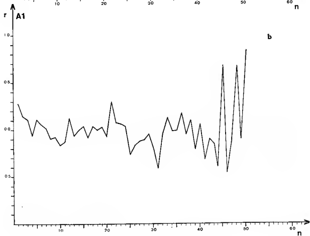
FIG. 51. --- Graphe d'autocorrélation de Phryganella ceropodia dans la peissière, a : individus vivants ; b : individus enkystés.
