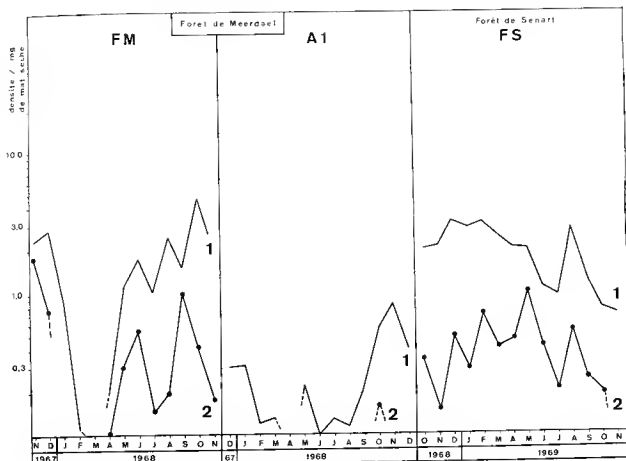
Fig. 62. — Densités moyennes mensuelles d' Euglypha rotunda : thèques vides (1) individus vivants (2) dans les trois stations.
