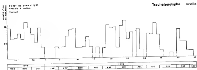
Fig. 63. — Densités hebdomadaires de Tracheleuglypha acolla dans la chênaie à molinie.
