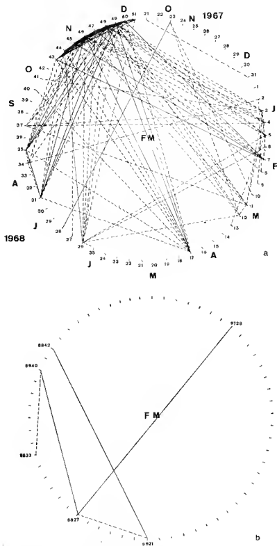
FIG. 79. — a : Noyaux d'affinités entre les relevés hebdomadaires dans la chénaie à luzule, b : dissimilarités entre les relevés hebdomadaires dans la chénaie à luzule.
