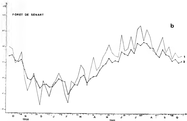
FIG. 6. — a : Températures maximales et minimales moyennes hebdomadaires en Forêt de Sénart, b : températures moyennes hebdomadaires de l'air (1) et du sol à -5\text{ cm} (2) en Forêt de Sénart.
