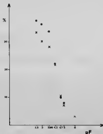
FIG. 4. — Potentiel capillaire, × : chénaie à luzule, 0 : pessière.
