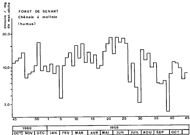
FIG. 30. — Densités hebdomadaires du peuplement de la chênaie à mollinie (d'après Coûtreaux, 1975 a).
