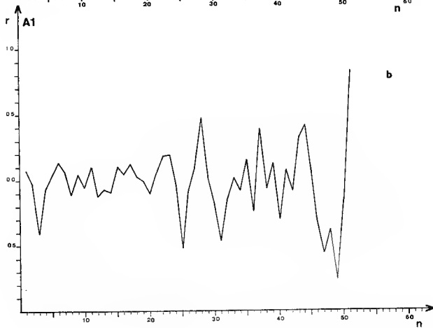
FIG. 40. — Graphe d'autocorrélation de Plagiopyxis declivis , a : châtaigne à luzule, b : pessière.
