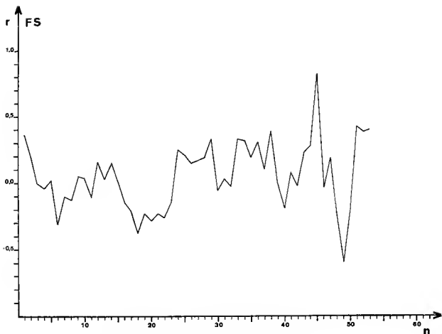
FIG. 65. — Graphé d'autocorrélation de Tracheleuglypha acolla dans la chénaie à molinie (d'après COÛTEAUX, 1975 a).
