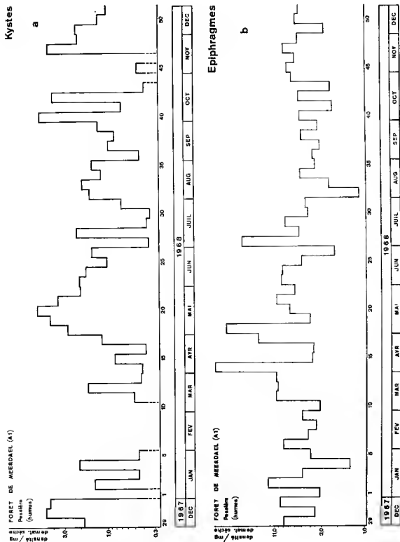
FIG. 27. — Densités hebdomadaires dans la pestière, a : individus enkystés, b : individus enkystés, b : individus dont la thèque est munie d'un épiphragme.
