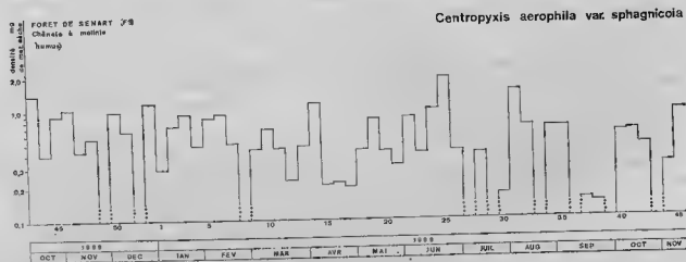
FIG. 35. Densités hebdomadaires de Centropyxis aerophila var. sphagnicola dans la chénaie à molinie.
