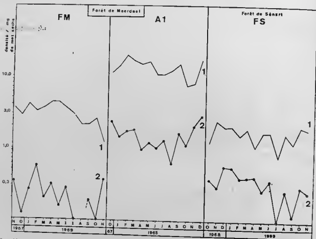
FIG. 43. — Densités moyennes mensuelles de Trigonopyxis arcua : thèque vides (1), individus vivants (2), dans les trois stations.
