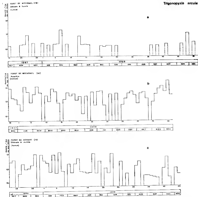
FIG. 42. — Densités hebdomadaires de Trigonopyxis arcuata , a : dans la chênaie à luzule, b : dans la pessière, c : dans la chênaie à molinie.
