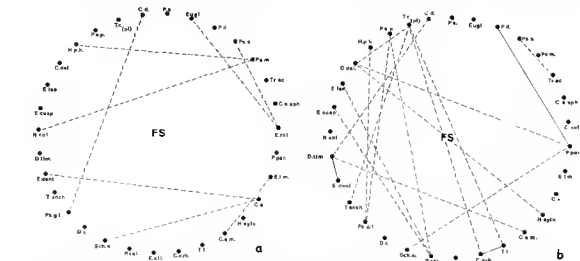
FIG. 88. — a : Noyau d'affinités entre les 31 espèces principales de la chénaie à molinie, b : dissemblances entre les 31 espèces principales de la chénaie à molinie.
