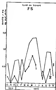
FIG. 47. — Densités moyennes mensuelles de Schoenbornia visciicola , dans la chênaie à molinia.
