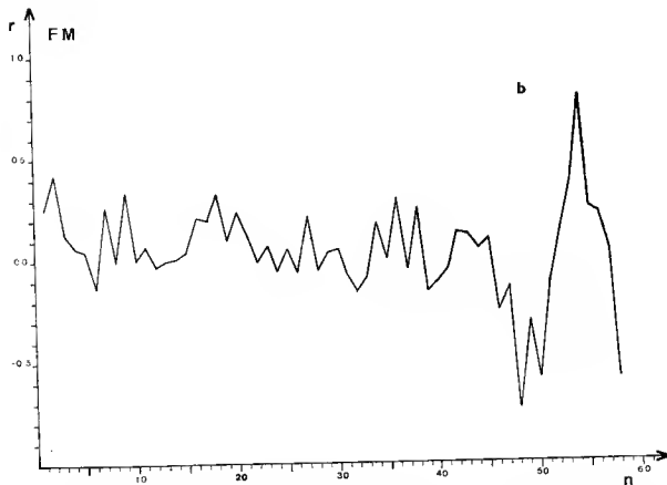
FIG. 24. — Graphe d'autocorrélation dans la chénaie à luzule, a : individus vivants (d'après COÛTEAUX, 1975 a) ; b : thèque vides.
