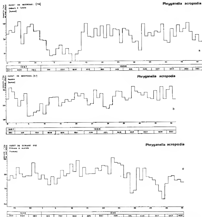
Fig. 48. — Densités hebdomadaires de Phryganella acropodia , a : dans la chênaie à luzerne, b : dans la pessière, c : dans la chênaie à molinie.
