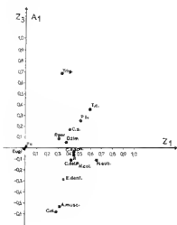
FIG. 87. — Représentation graphique des 16 espèces principales de la peissière en fonction de leur saturation en premier et troisième facteurs.
