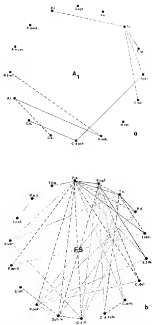
FIG. 86. — Noyaux d'affinités, a : entre les 16 espèces principales de la peillère, b : entre les 18 espèces les plus abondantes de la chénaie à molinie.
