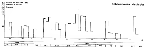
FIG. 46. — Densités hebdomadaires de Schoenbornia visciicola dans la chênaie à molinia.
