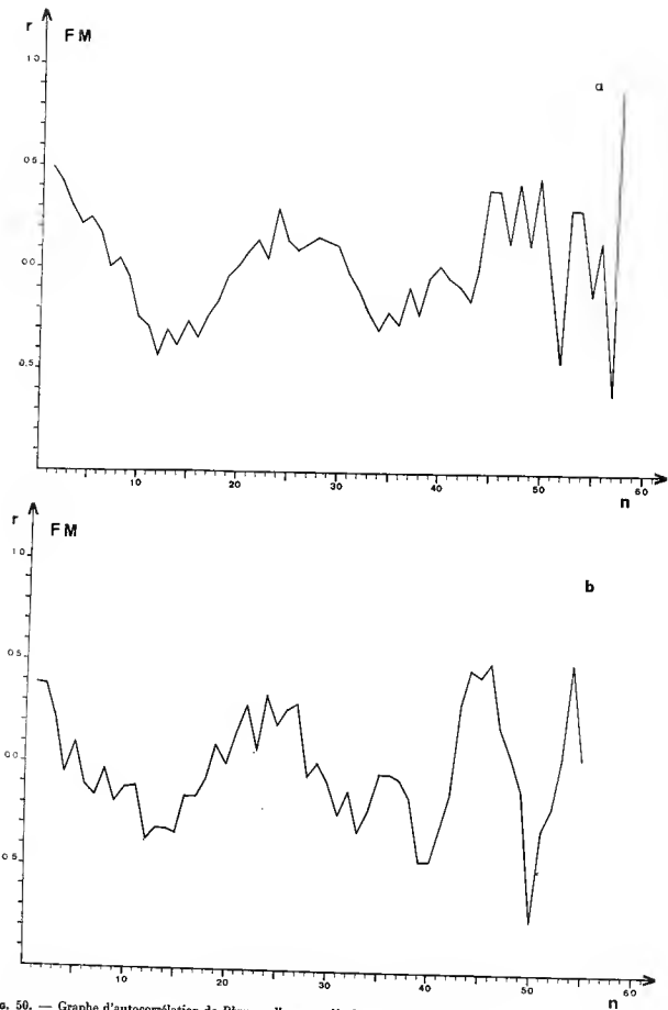
FIG. 50. — Graphe d'autocorrélation de Phryganella acropodia dans la chênaie à luzule, a : individus vivants ; b : individus enkystés.
