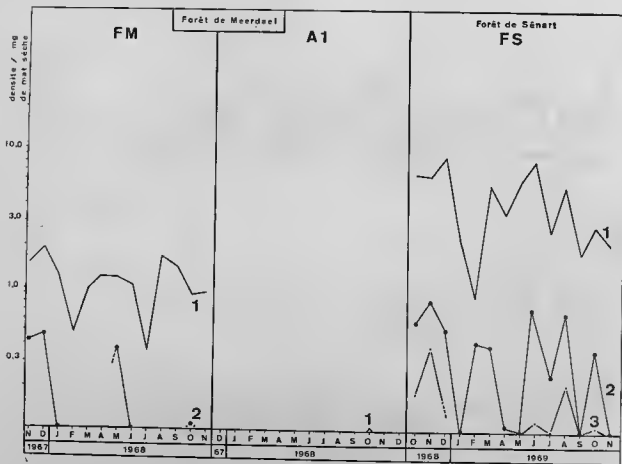
Fig. 66. — Densités moyennes mensuelles de Tracheleuglypha acolla : thèques vides (1), individus vivants (2) dans les trois stations.
