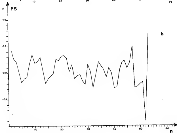
FIG. 33. — Graphe d'autocorrélation dans la chénaie à molinie, a : individus enkystés ; b : individus dont la thèque est munie d'un épiphragme (d'après COÛTEAUX 1975 a).
