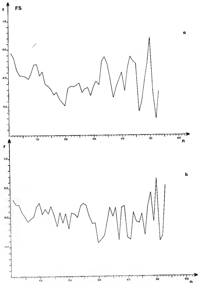
FIG. 32. — Graphe d'autocorrélation dans la chênaie à molinie, a : individus vivants (d'après COÛTEAUX, 1975 a) ; b : théques vides.
