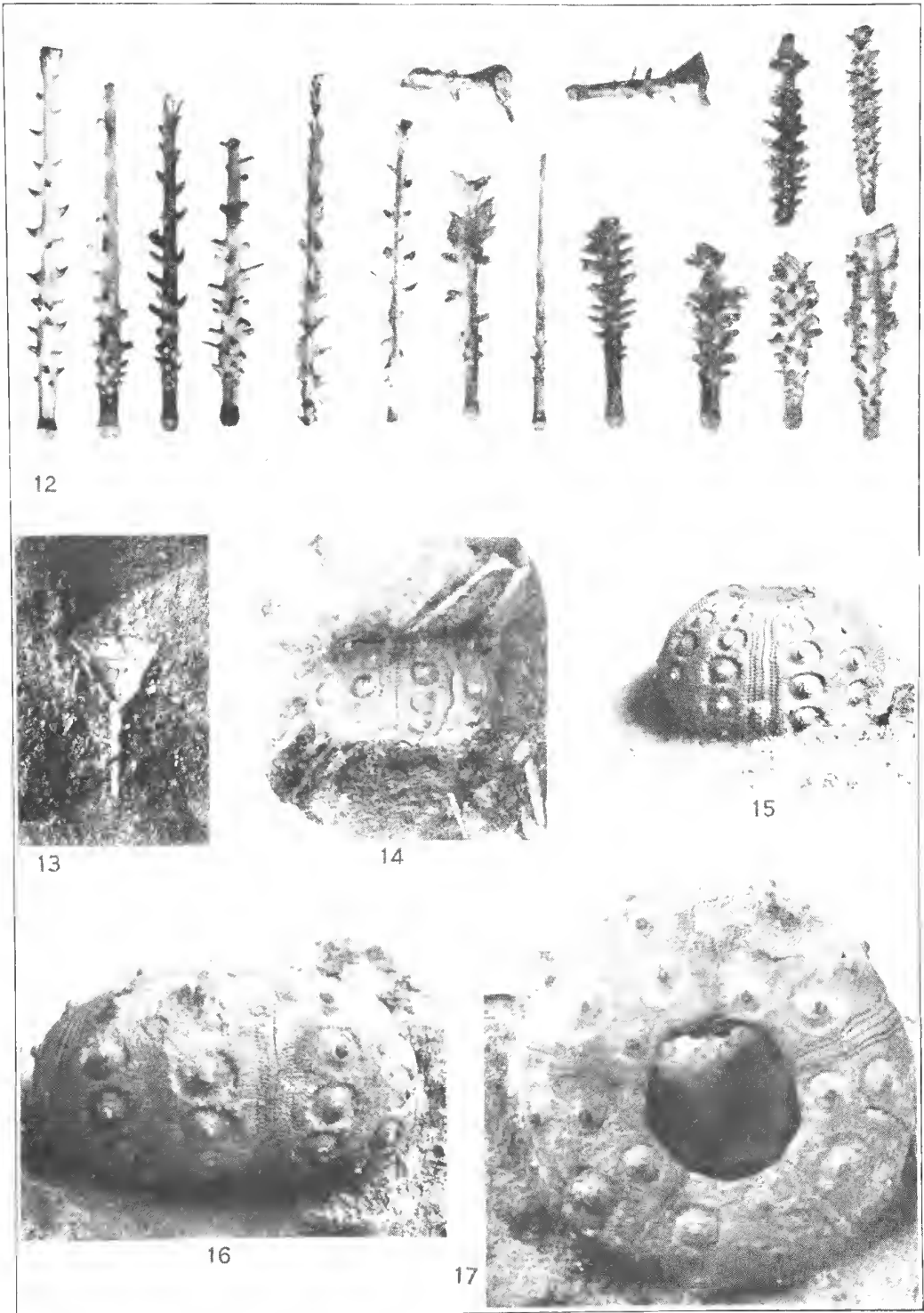
Cainozoic Cidaroids
