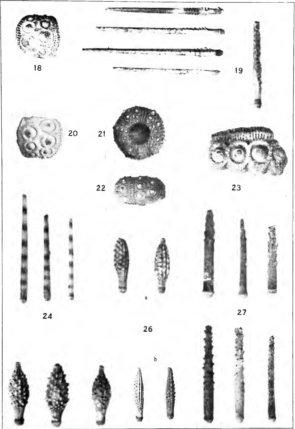
Cainozoic Cidaroids
