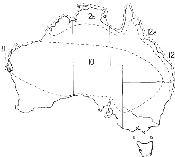
FIG. 3.—DISTRIBUTION.
