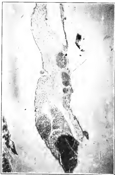
FIG. 3—PODANOMYUS.
