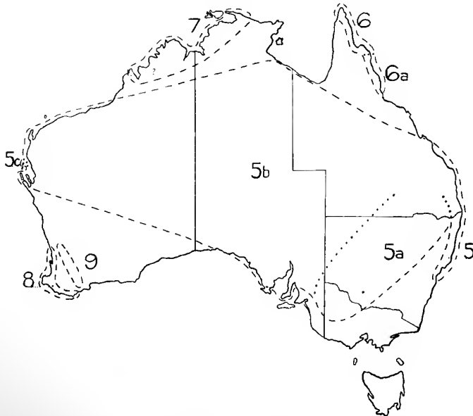
FIG. 2—DISTRIBUTION.
