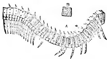
Fig. 8. Euphoberia granosa .
