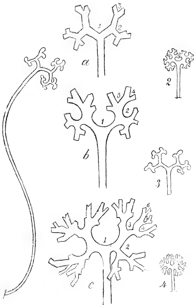
a, b, c, 1 a , 2 a y 3 a : fase del desarrollo de una tufa de la Micosphaera sophorae (nuev. esp.). (Muy aumentadas y tomadas con cámara clara).— 1, Apendículo de la M. Guarinonii .—2, Id. de la M. alni ó penicillata . —3, Id. de la M. loniceræ .—4, Id. de la M. grossulariæ .
