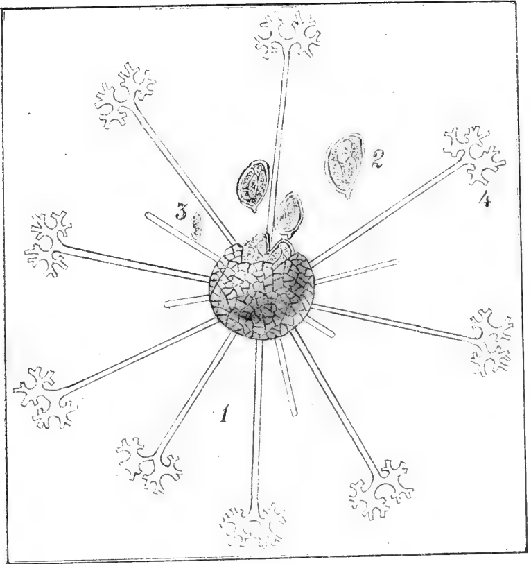
Fig. 1.— Microsphaera sophorae (nuev. esp.) 1, Periteca en general.—2, Asca.—3, Espora.—4, Apendículo con su tufa
