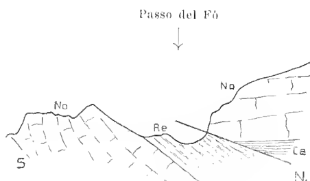
Fig. 9. — Profilo attraverso il Passo del Fò. (Ca = Carnico; No = Norico; Re = Retico).
