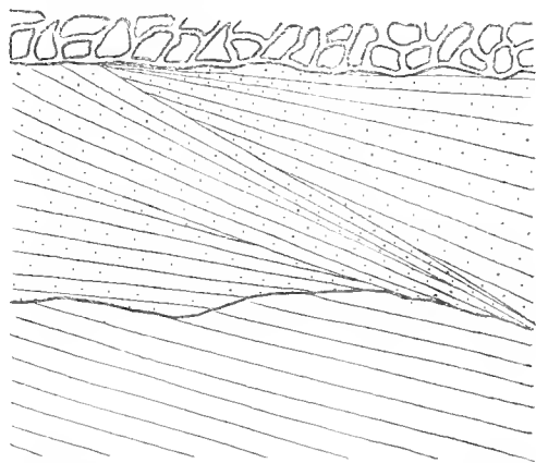
Fig. 6. — Discordanza nel Pliocene del Torrente Tornago presso Almenno.
