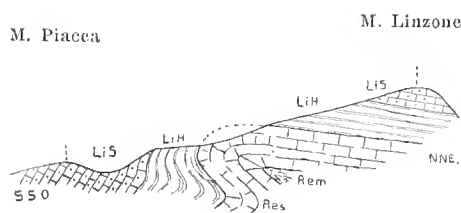
Fig. 12. — Profilo attraverso il fianco meridionale del M. Linzone. (Rem = Retico medio; Res = Retico superiore; LiH = Hettangiano; LiS = Sinemuriano).
