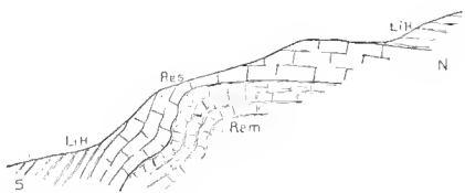
Fig. 13. — La piega dell'Albenza in Val di Malanotte. Schizzo dal vero. (Per le abbreviazioni cfr. fig. 12).
