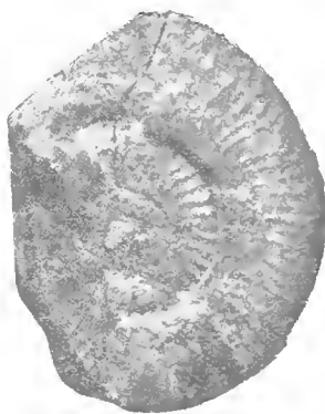
Fig. 27. — Hildoceras Emilianum Reyn. Esemplare dei dintorni di Almenno (Lias sup.).
