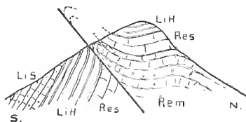
Fig. 15. — Profilo attraverso « il Botto ». (Per le abbreviazioni cfr. fig. 12).
