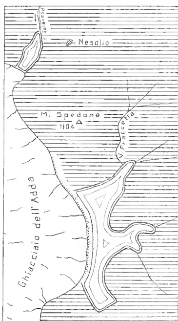
Fig. 7. — Ricostruzione dei due laghi singlaciali di Carenno e di Erve. Scala 1:50000.
