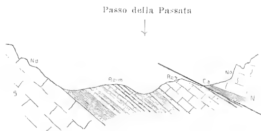
Fig. 10. — Profilo attraverso il Passo della Passata. (Ca = Carnico; No = Norico; Reim = Retico medio e inferiore; Res = Retico superiore).
