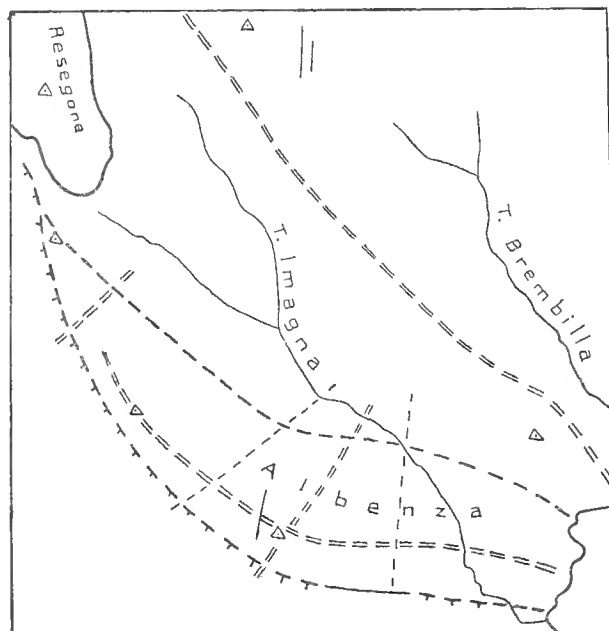
Fig. 22. — Schizzo tettonico del gruppo dell'Albena. Scala: 150.000. (- + anticlinali. La sbarretta indica la direzione in cui sono inclinate. == sinclinali. ———— margini della falda del Resegone. ———— faglie).
