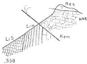
Fig. 14. — Profilo attraverso il fianco meridionale della Corna Rocchetto. (Per le abbreviazioni cfr. fig. 12).
