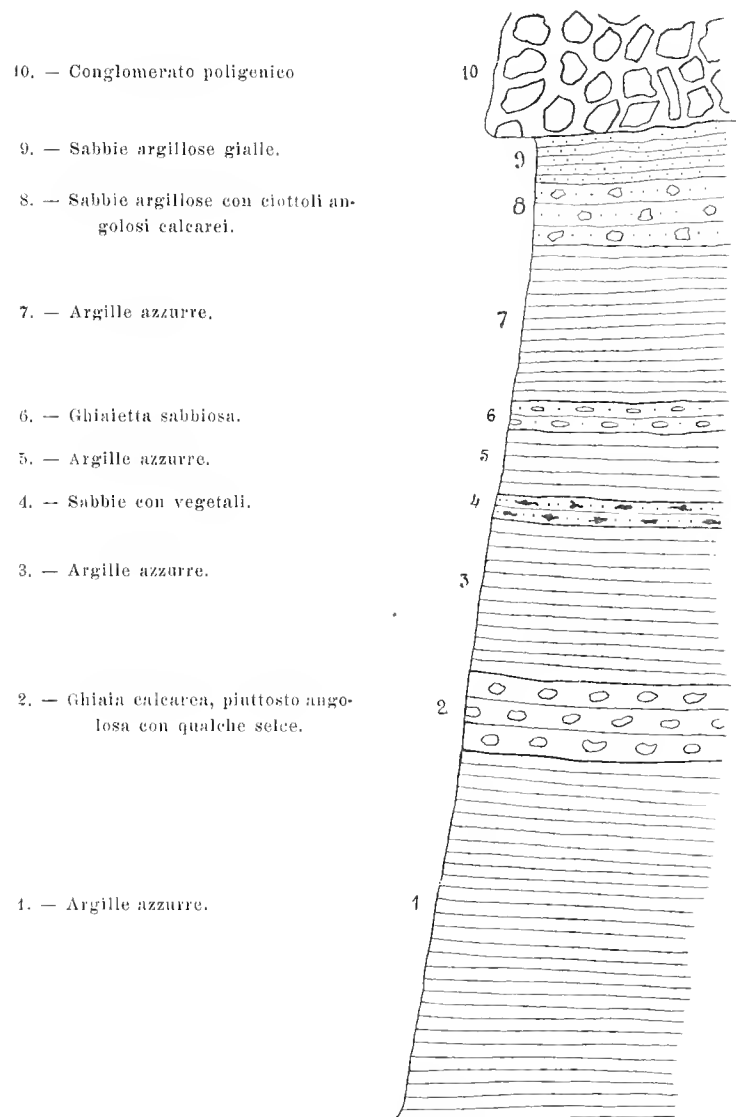
Fig. 5. — Profilo nel lembo pliocenico del Torrente Tornago presso Almenno (Scala 1:50).
