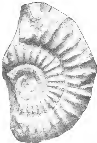
Fig. 24. — Arietites ( Arnioceras ) mendax var. rariplacatum Fuc. Esemplare dei dintorni di Carenno (Lias. inf.)
