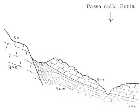
Fig. 11. — Profilo attraverso il Passo della Porta. (No = Norico; Rem = Retico medio; Res = Retico superiore).
