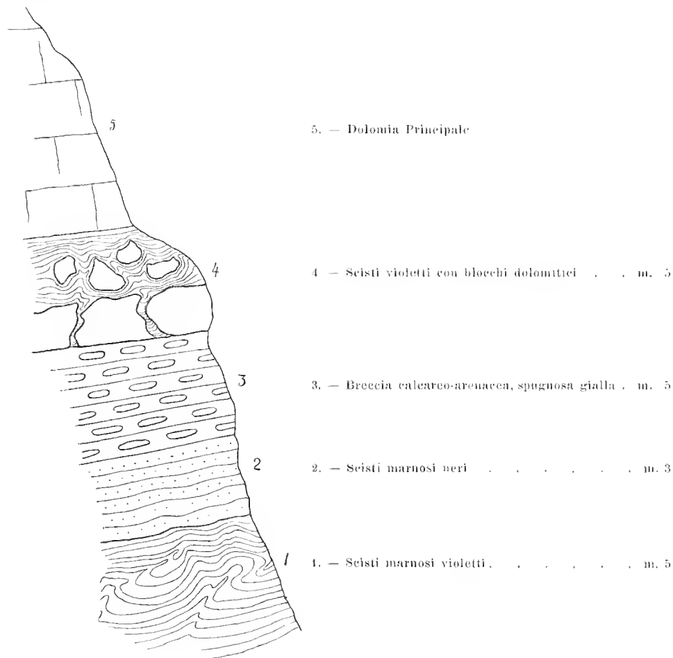
Fig. 1. — Sezione naturale presso la Cap. Alpinisti Monzesi in Val d'Erve.
