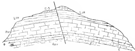
Fig. 21. — Una delle faglie dei « Canti ». (Per le abbreviazioni cfr. fig. 18).
