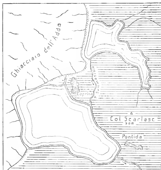
Fig. 8. — Ricostruzione dei due laghi singlaciali di Cisano e di S. Antonio d'Adda. Scala 1:50000.
