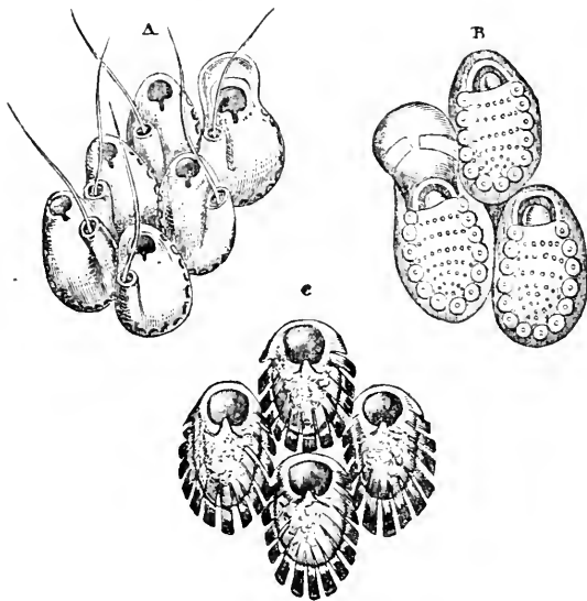
Cells of Lepralica :—A, L. Hyndmanni ; B, L. figularis ; C, L. verrucosa .
