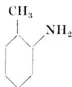
Toluidine (ortho)
