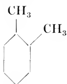
Xylene (ortho)
