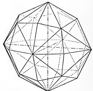
FIG. 73.—The Hexahedron, 3a : a : 2a .
