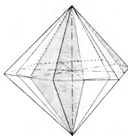
FIG. 191. — The Plus Ditrigonal Pyramid ( hk\bar{i}l ).
