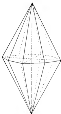
FIG. 113.—The Ditetragonal Pyramid.
