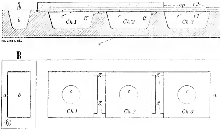
Fig. 1. — Nid artificiel en substance poreuse (plâtre, terre éuite, pierre tendre, etc.). B, Vue du nid en plan. La plaque opaque destinée à maintenir l'obscurité est supposée enlevée; A, coupe verticale.
