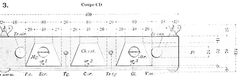
APPAREIL POUR L'OBSERVATION DES FOURMIS ET DES ANIMAUX MYRMÉCOPHILES.
